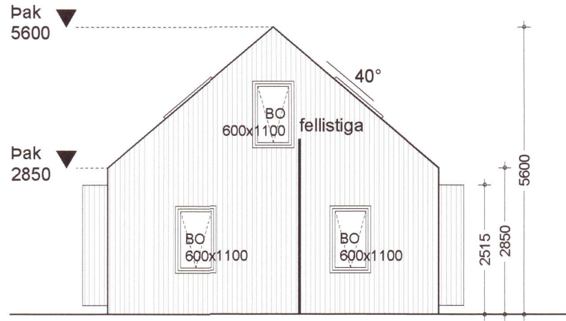
Ásýnd norður
