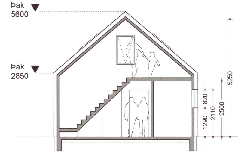
Skurðmynd B-B
