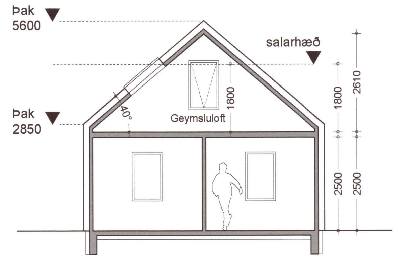
Skurðmynd A-A
