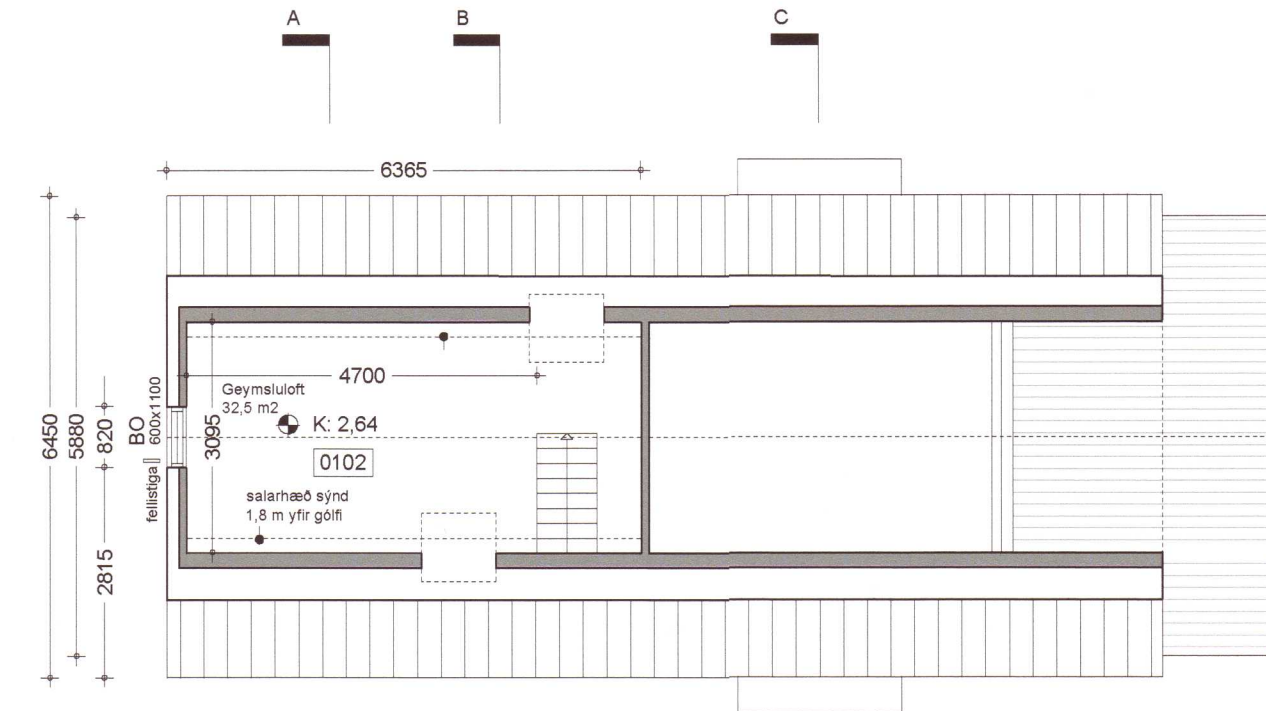
MHL 01 Grunnmynd geymslu loft 1:100
