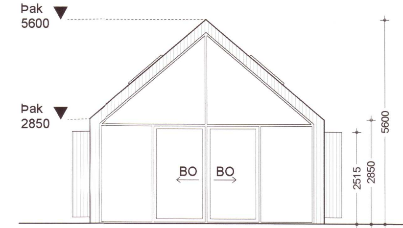
Ásýnd suður
