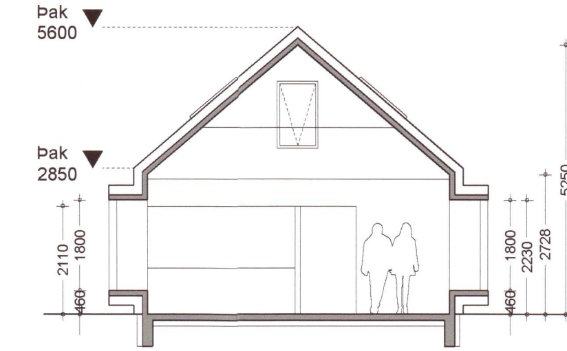
Skurðmynd C-C
