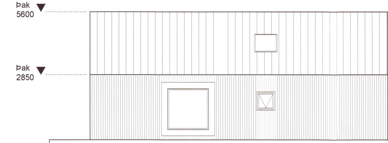
Ásýnd austur
