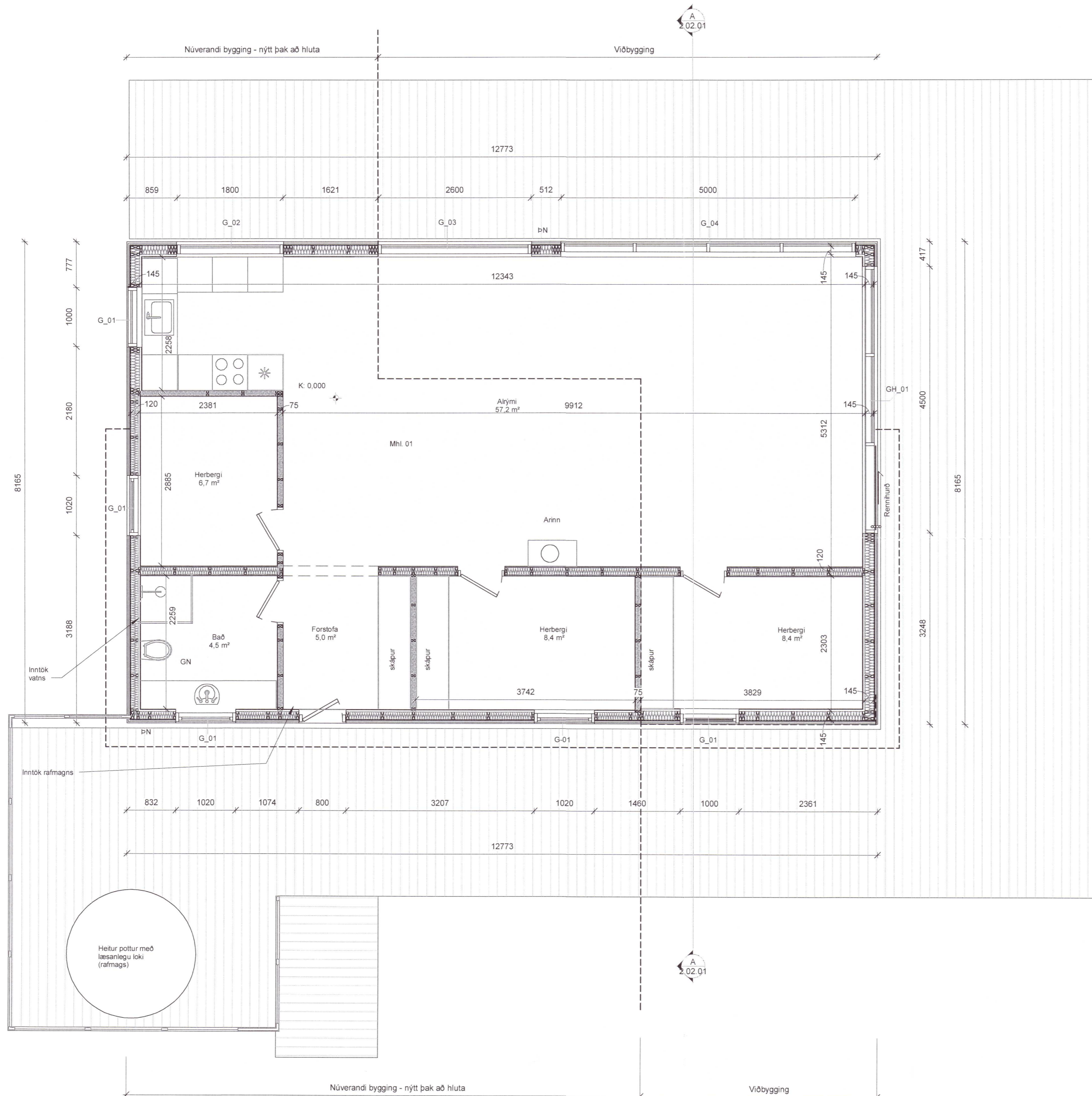
01- Grunnmynd_1_50 1 : 50
