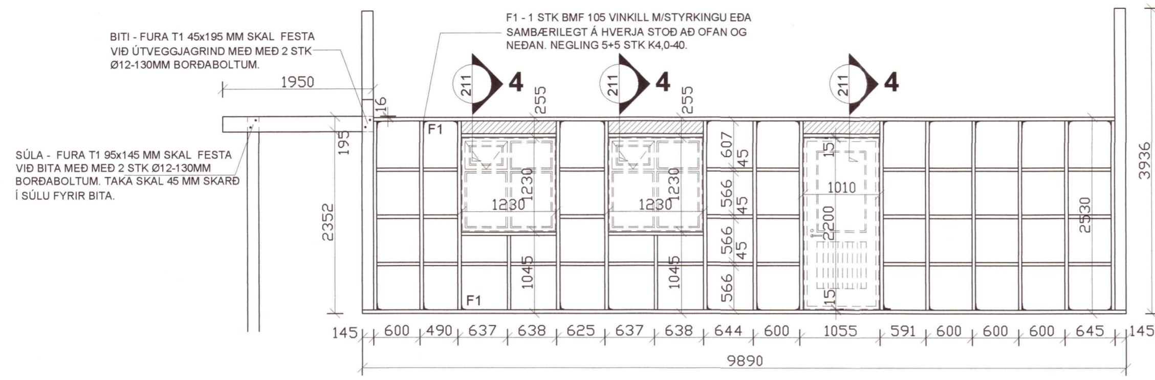
V4 - útlit - 1:50
