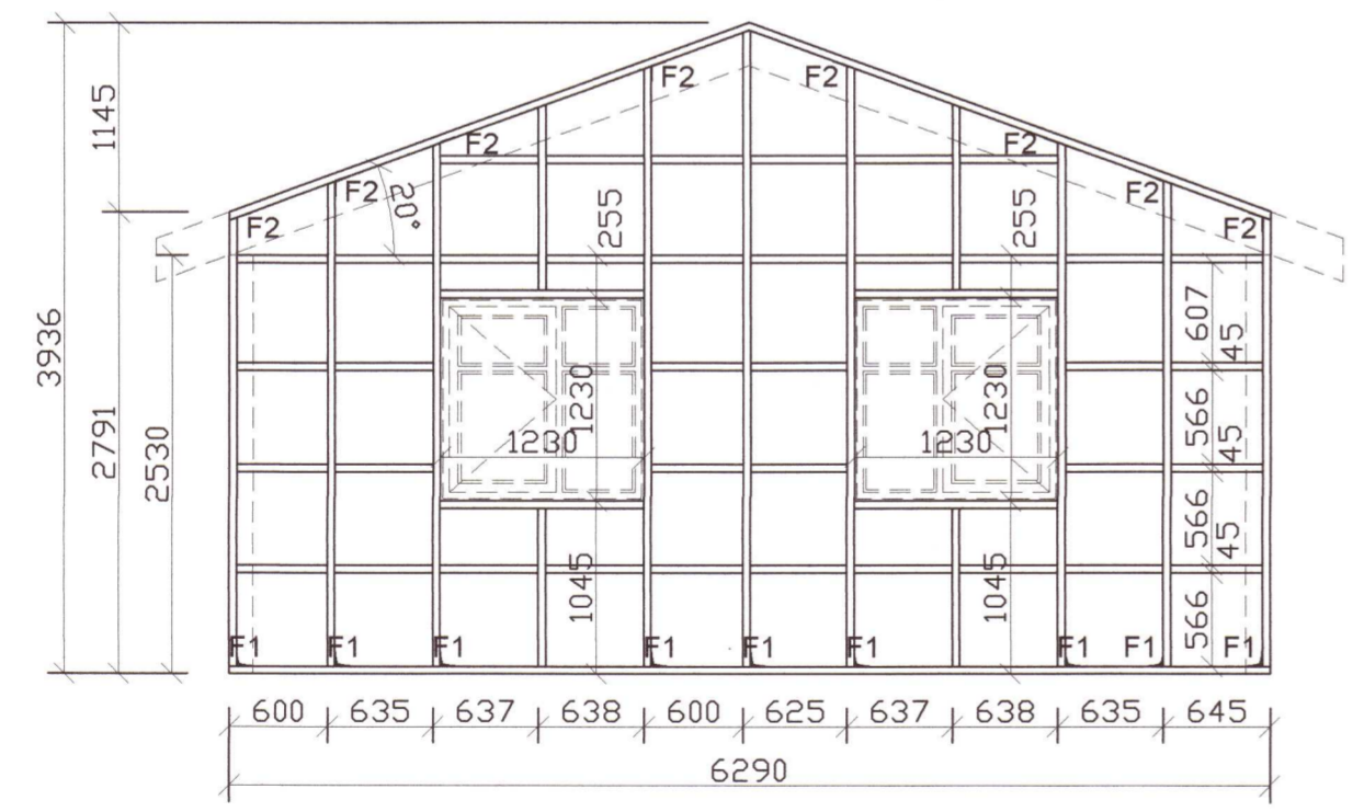
V3 - útlit - 1:50
