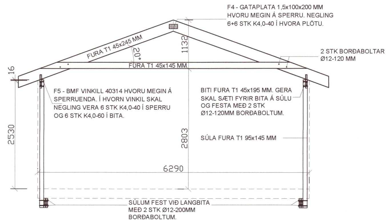
Snið 5 - 1:50
