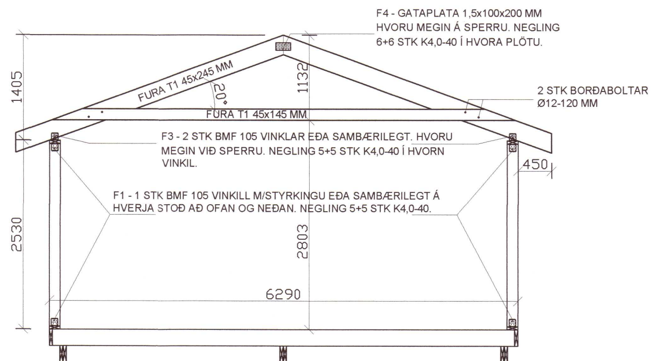
Snið 6 - 1:50
