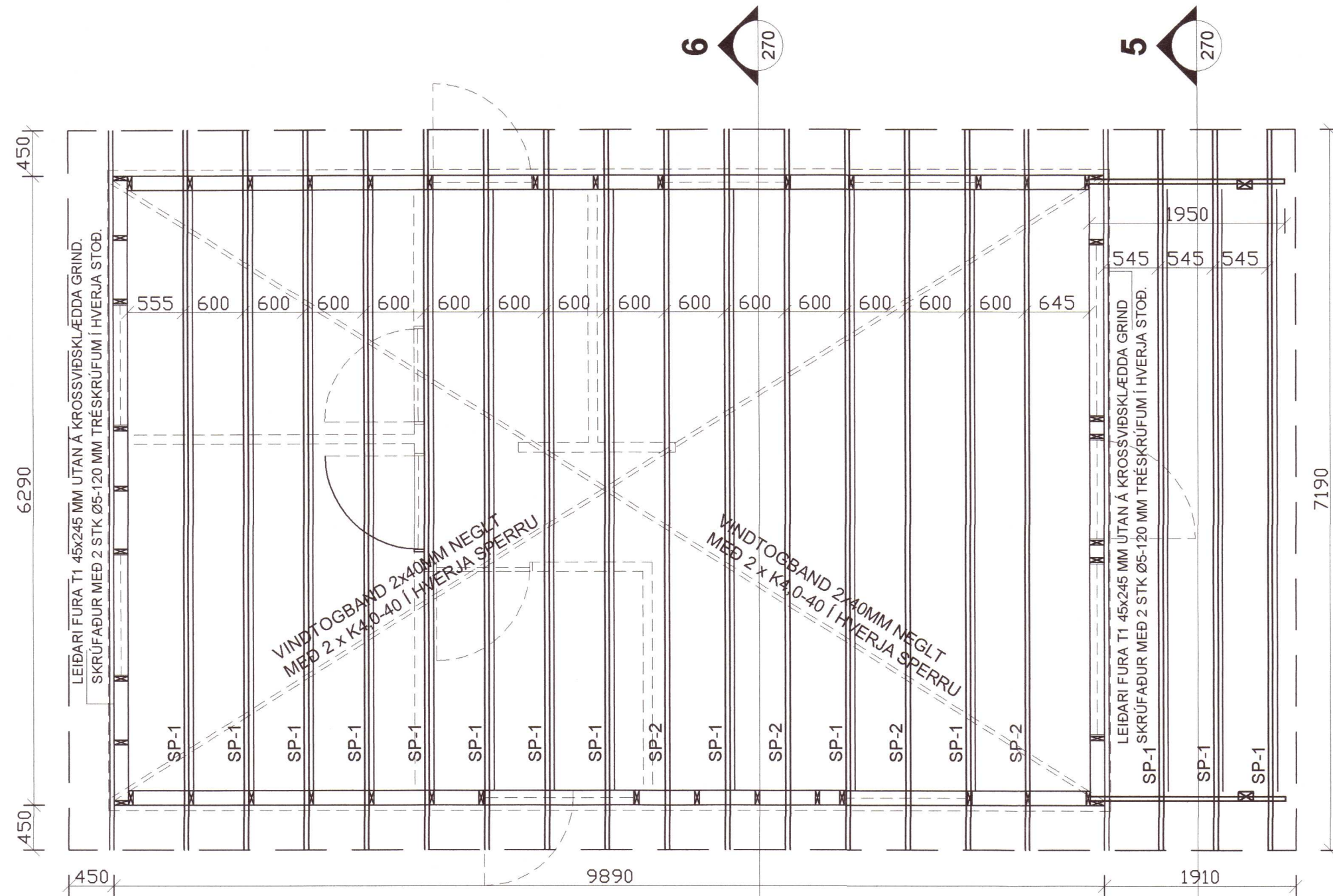
Grunnmynd - 1:50
