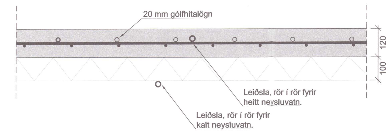
Frágangur lagna 1:10
