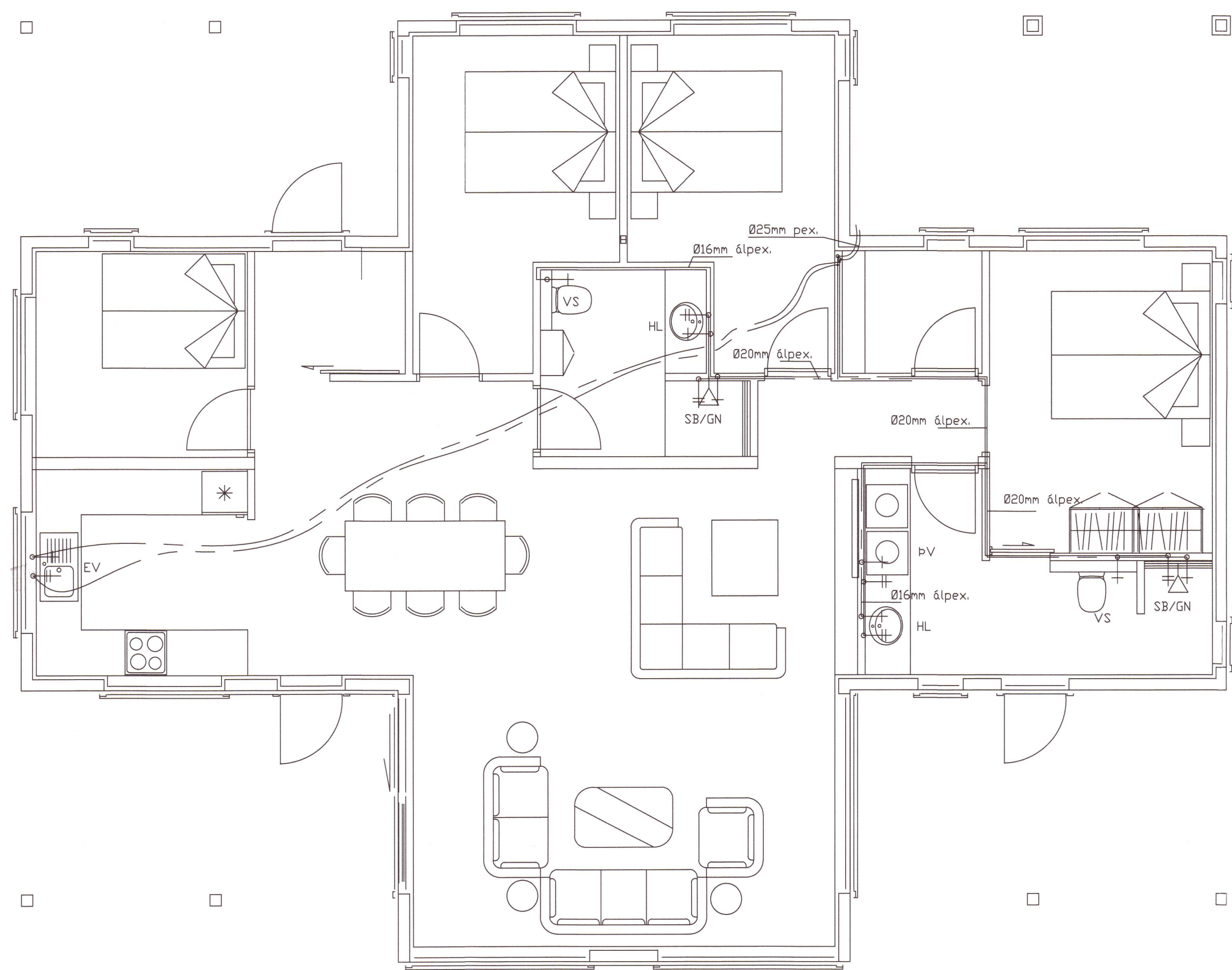
Grunnmynd Mkv. 1:50
