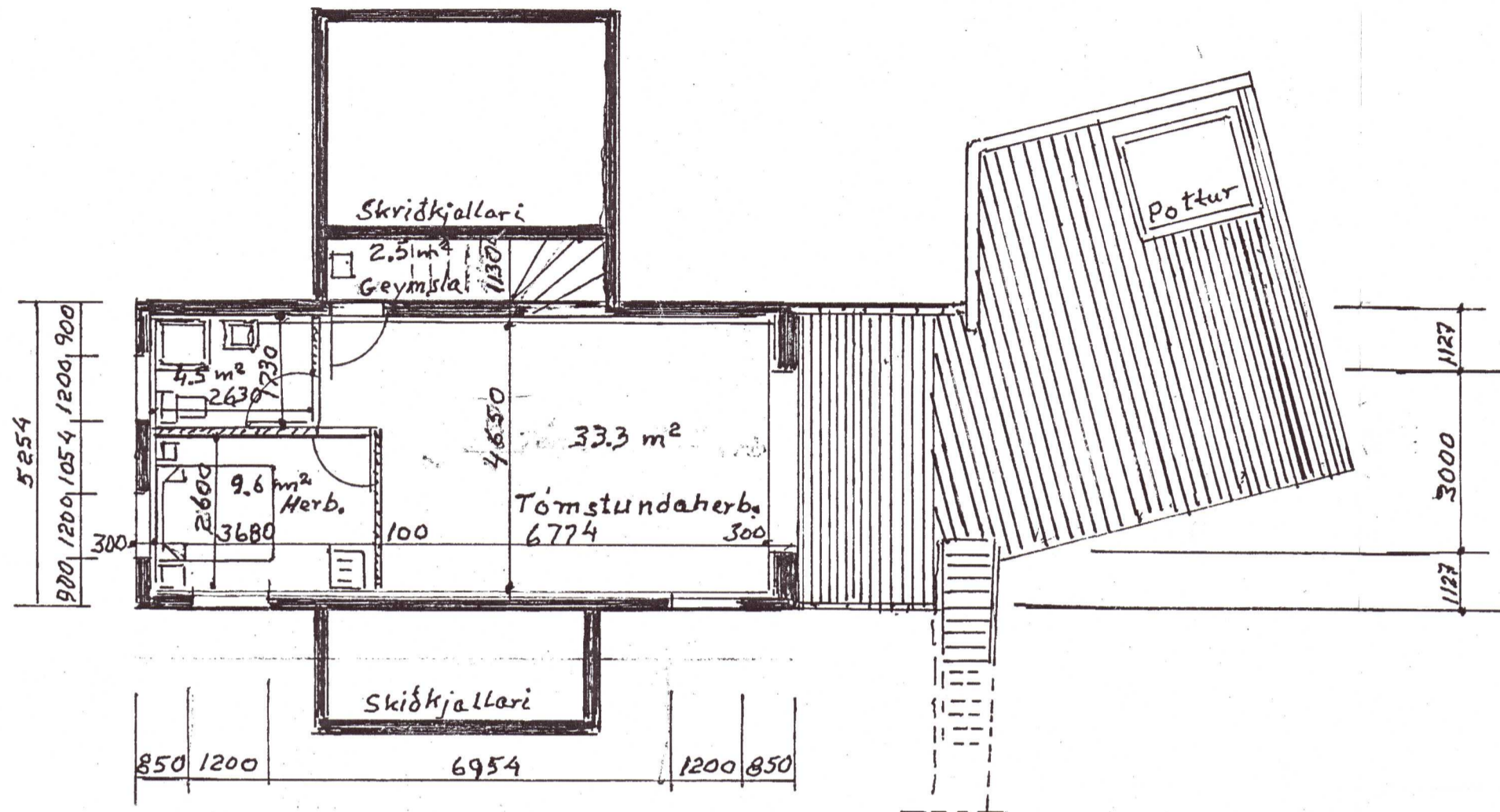
Kjallari, grunnmynd. M 1:100
