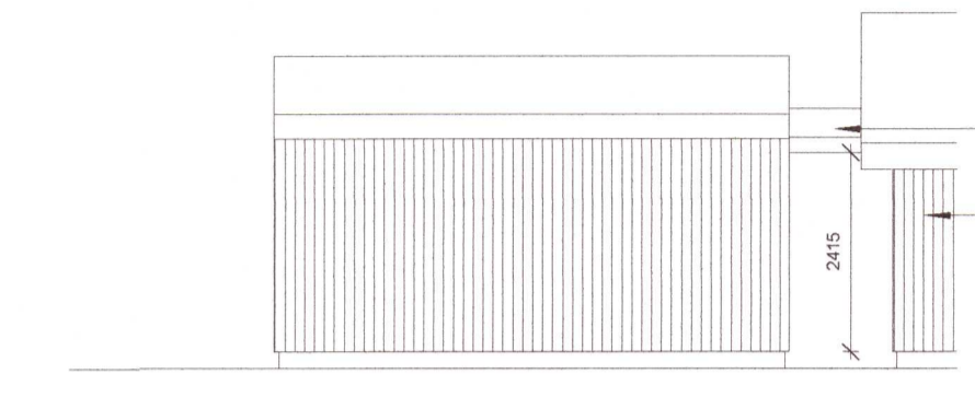
2 Austur 1:100
