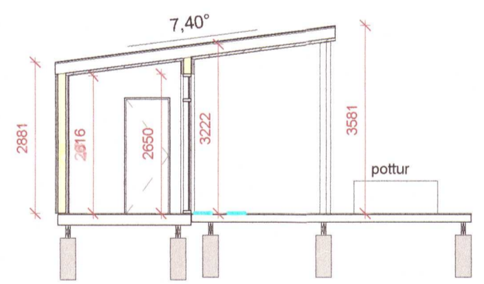
A Snið A-A 1:100
