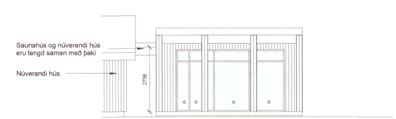
5 Vestur 1:100
