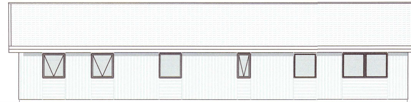
NORÐAUSTURHLIÐ
