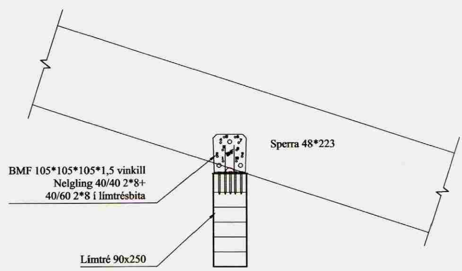
105 FESTING SPERRU VIÐ BITA YFIR ELDHÚSI 204/208 Mkv: 1/10
