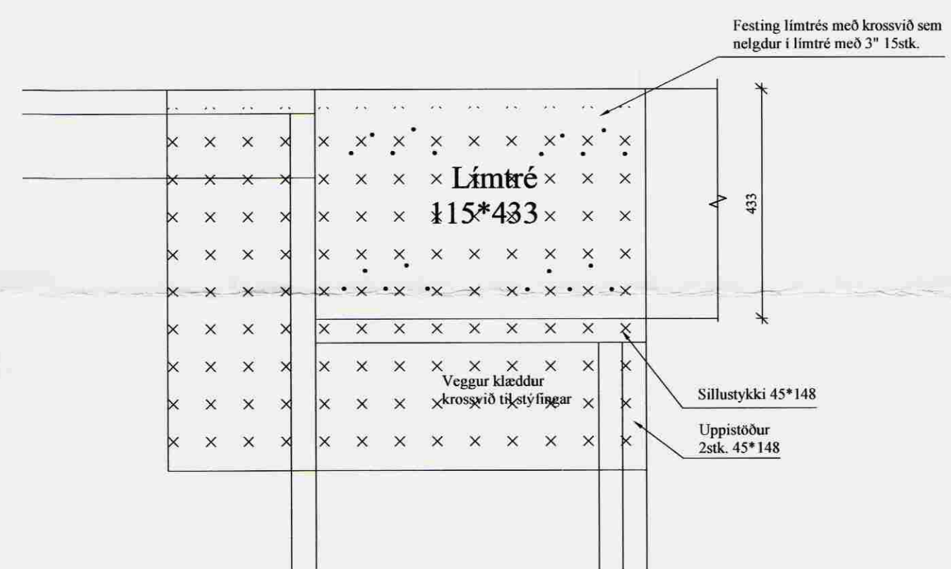
107 FESTING BITA VIÐ INNVEGG 204/208 Mkv: 1/10
