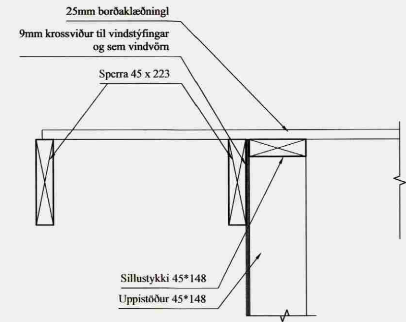
103 FRÁGANGUR VIÐ GAFLA 204/208 Mkv: 1/10
