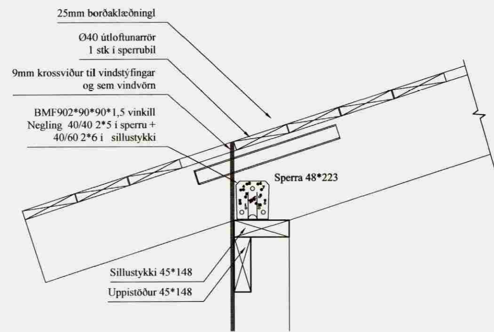
101 FESTING SPERRU VIÐ ÚTHLIDAR 204/208 Mkv: 1/10
