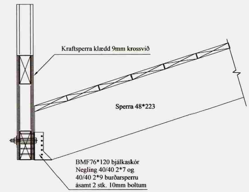
106 FESTING SPERRU VIÐ KRAFTSPERRU Í SUÐURHLUTA 204/208 Mkv: 1/10
