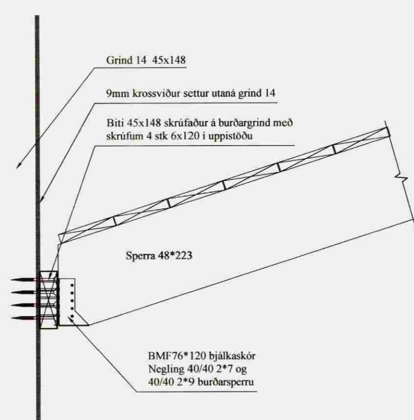
104 FESTING SPERRU VIÐ MILLIVEGG 204/208 Mkv: 1/10
