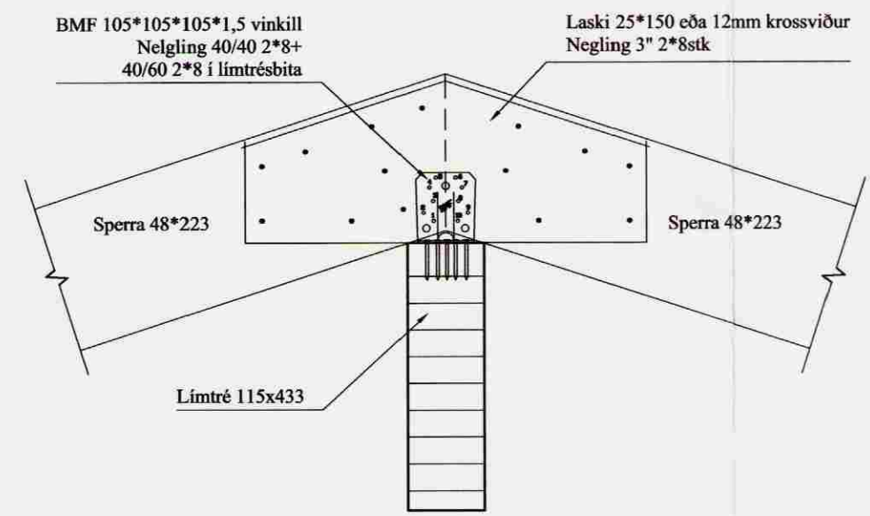
102 FESTING SPERRU Í MÆNI OG VIÐ BITA 204/208 Mkv: 1/10
