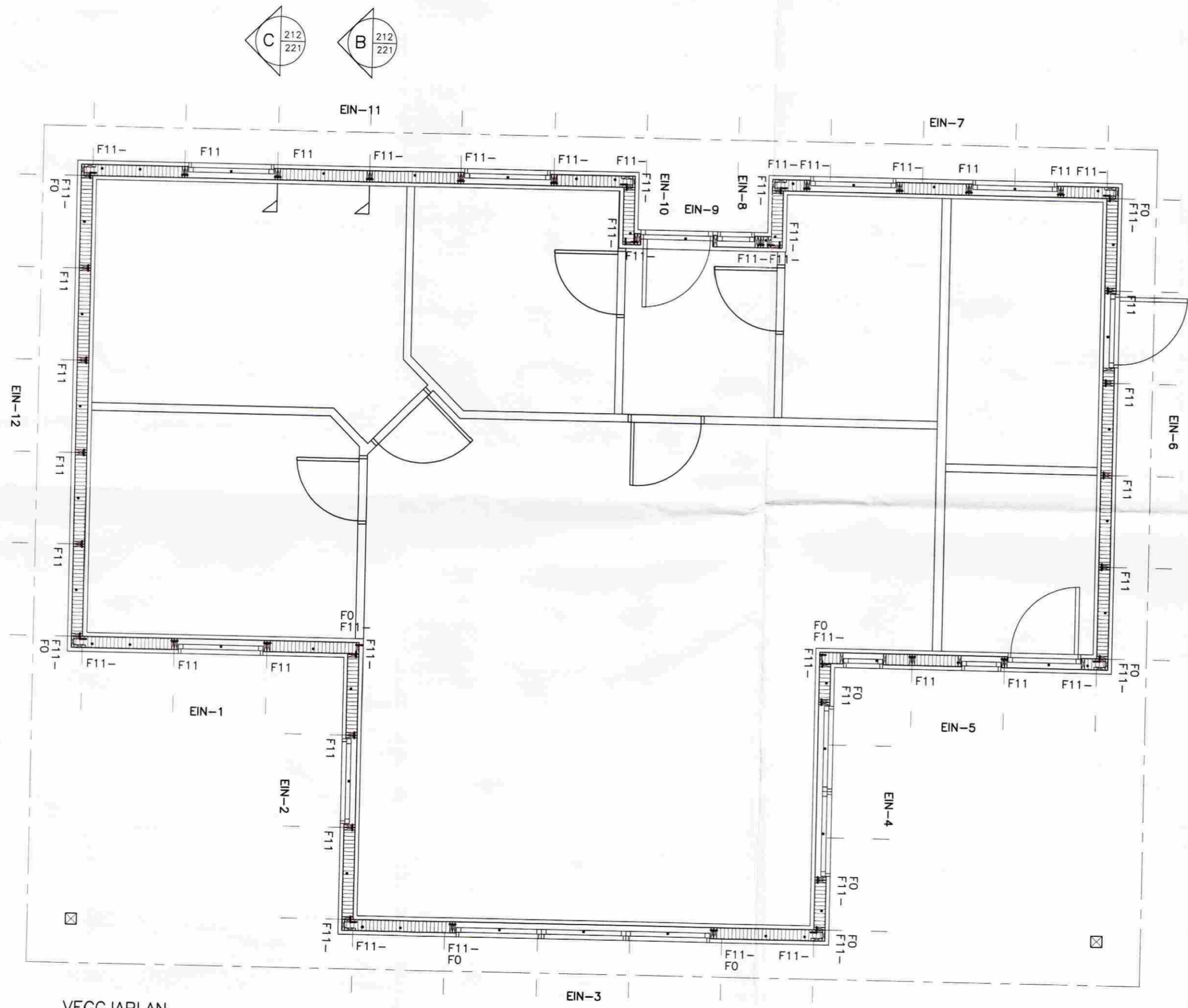
VEGGJAPLAN MKV. 1:50
