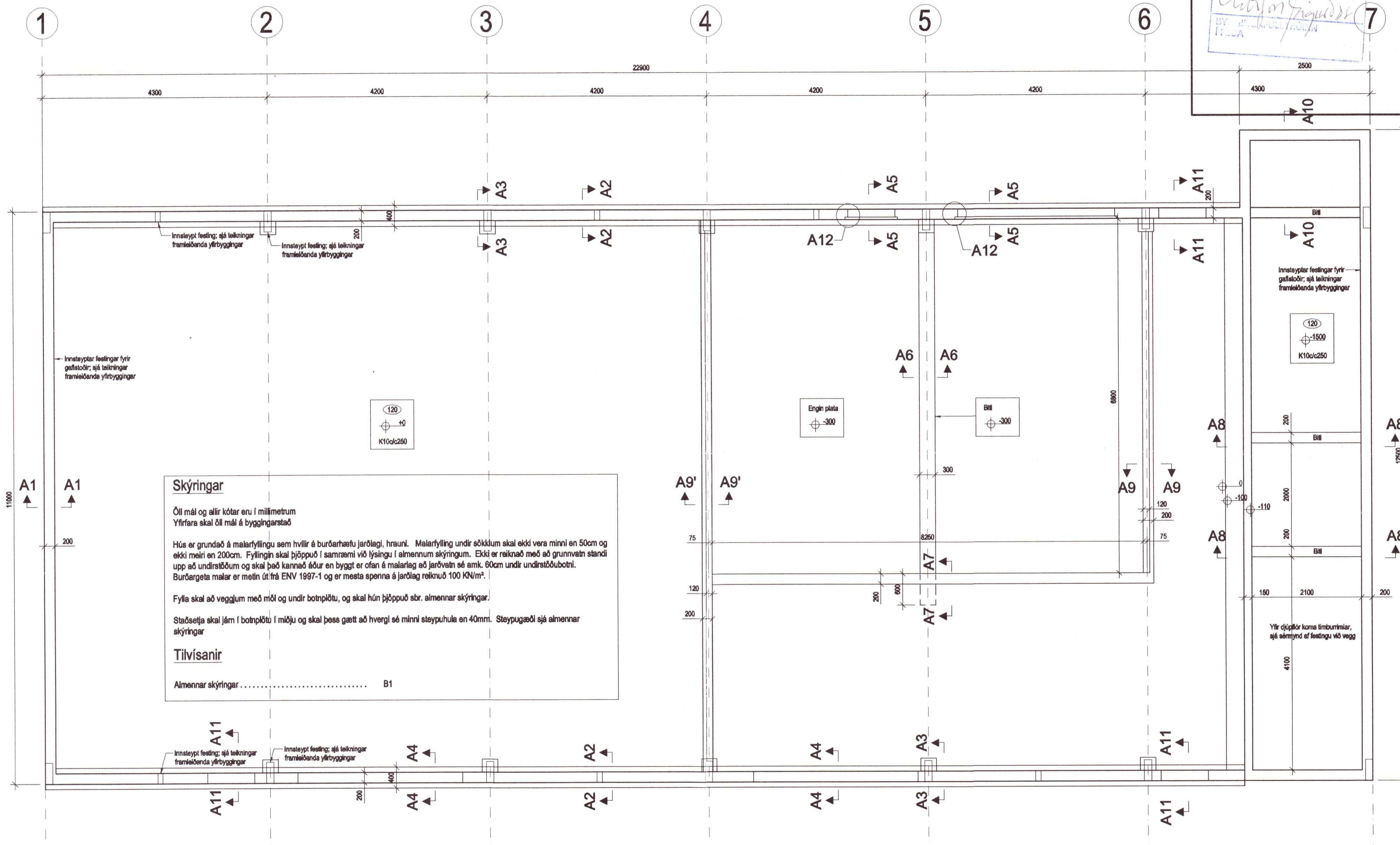
Undirstöður, grunnmynd 1:50
