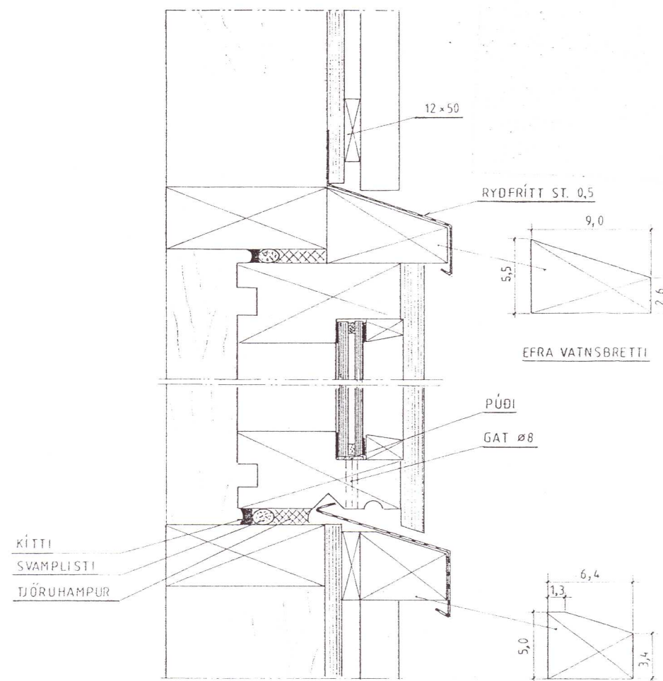
PVERSNIÐ Í GLUGGA MKV. 1:2
