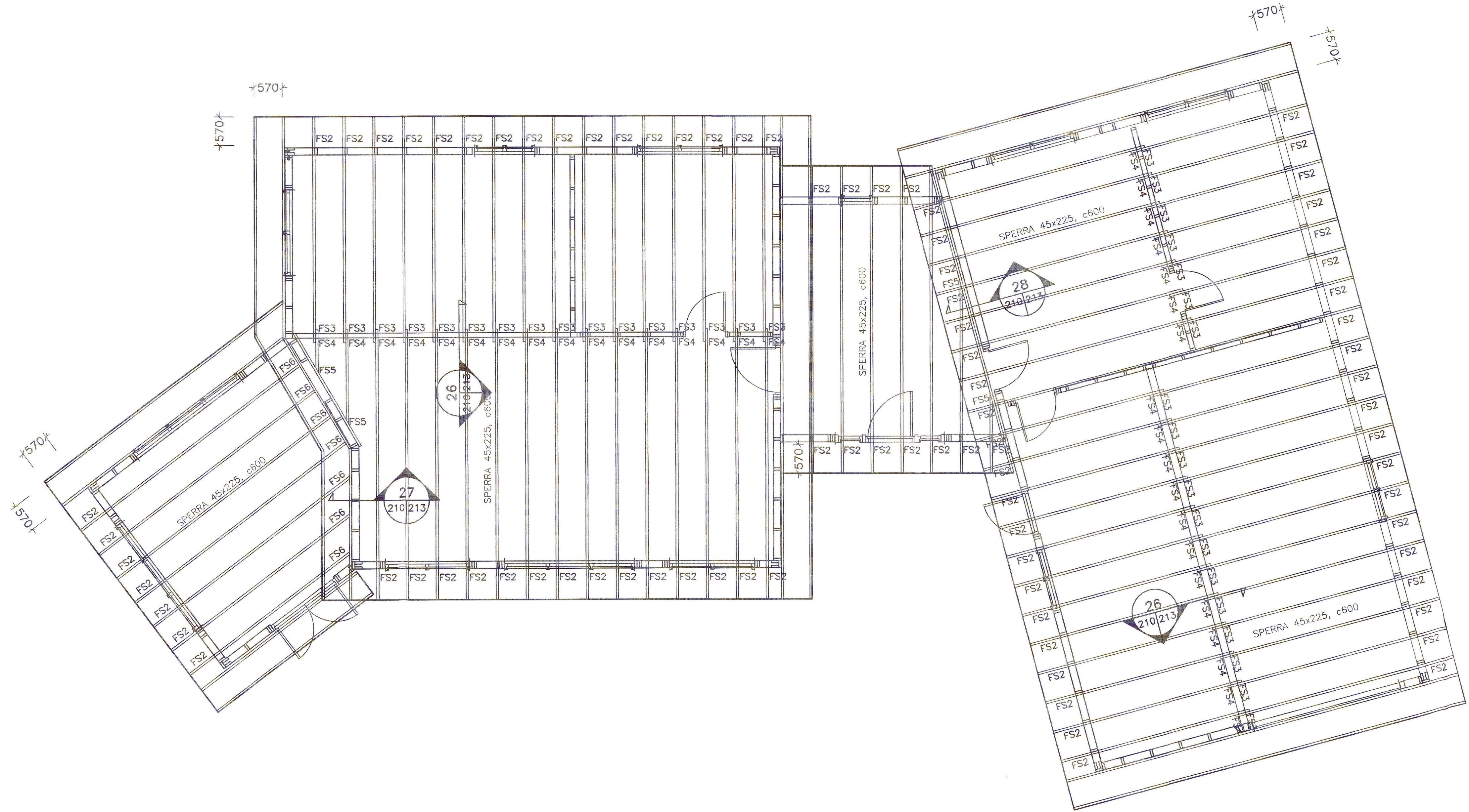
GRUNNMYND ÞAKPLAN MKV. 1
