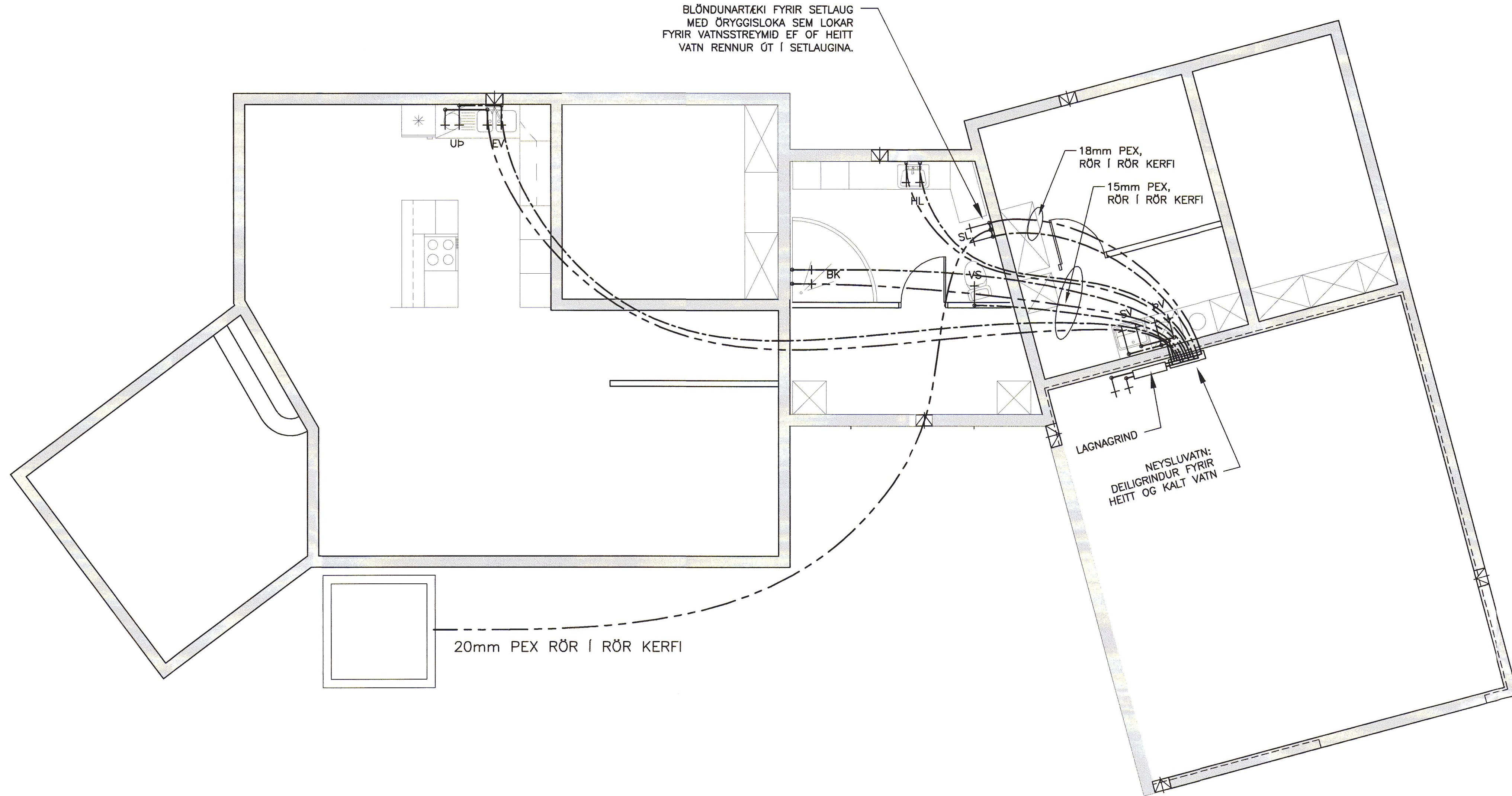
GRUNNMYND MKV. 1
