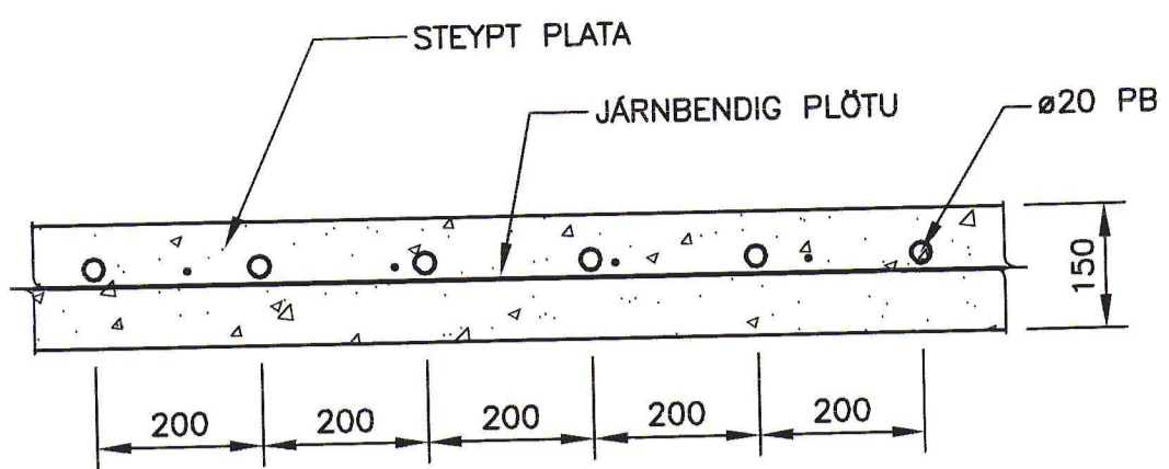
SNID Í GÓLFHITALÖGN Í STEYPTRI PLÖTU MKV. 2
