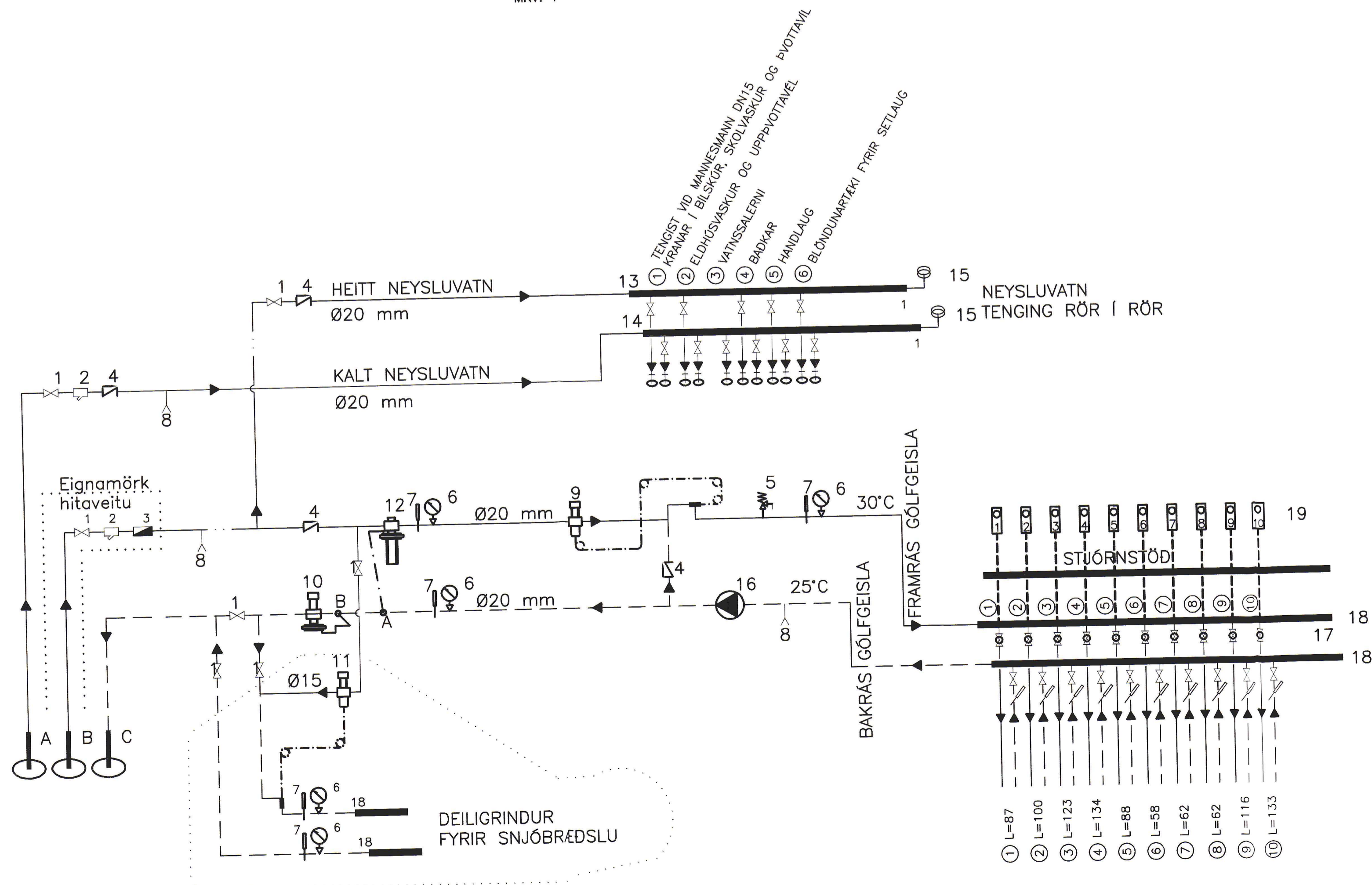
GRUNNMYND MKV. 1
