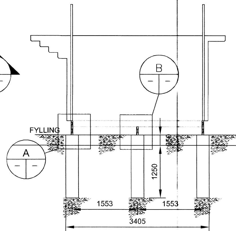
101 SNID MKV. 1
