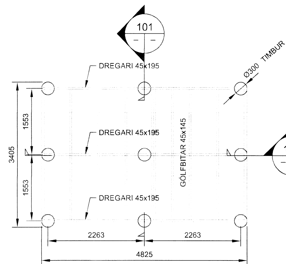
GRUNNMYND-UNDIRSTÖÐUR MKV. 1
