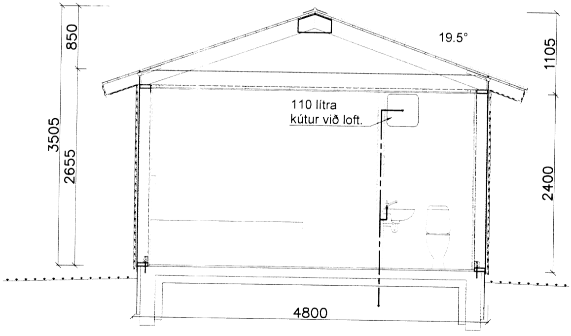
Snið Mkv. 1:50
