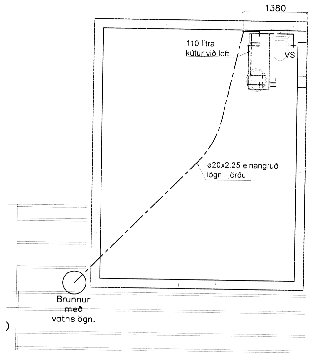
Grundmynd neysluvatnslagna Mkv. 1:50
