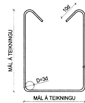
MYND II.3 - BEYGGING JÁRNA: OPIN LYKKJA
