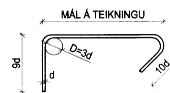
MYND II.4 - BEYGGING JÁRNA: NÆLUR
