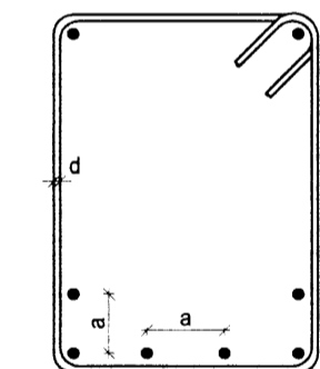
MYND II.5 - INNBYRÐIS FJARLÆGÐ JÁRNA
