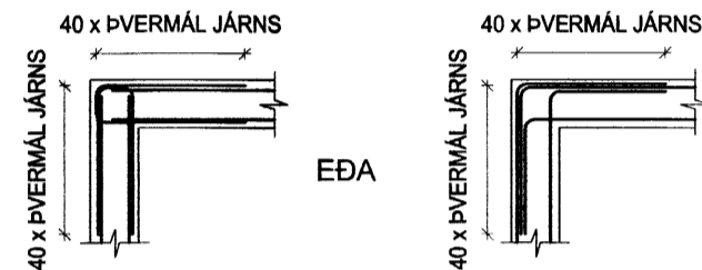
MYND II.9 - BENDING LÁRÉTTRA JÁRNA UM HORN
