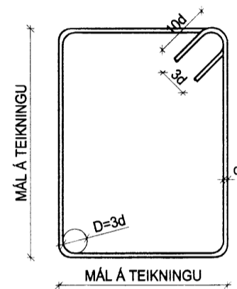
MYND II.2 - BEYGGING JÁRNA: LOKUÐ LYKKJA
