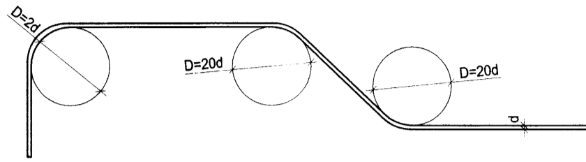
MYND II.1 - BEYGGING JÁRNA: UPPBEYGGJUJÁRN
