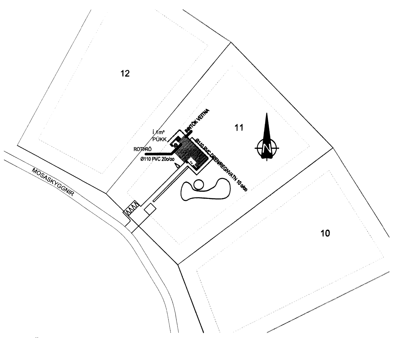
AFSTÖÐUMYND MKV. 1:1500
