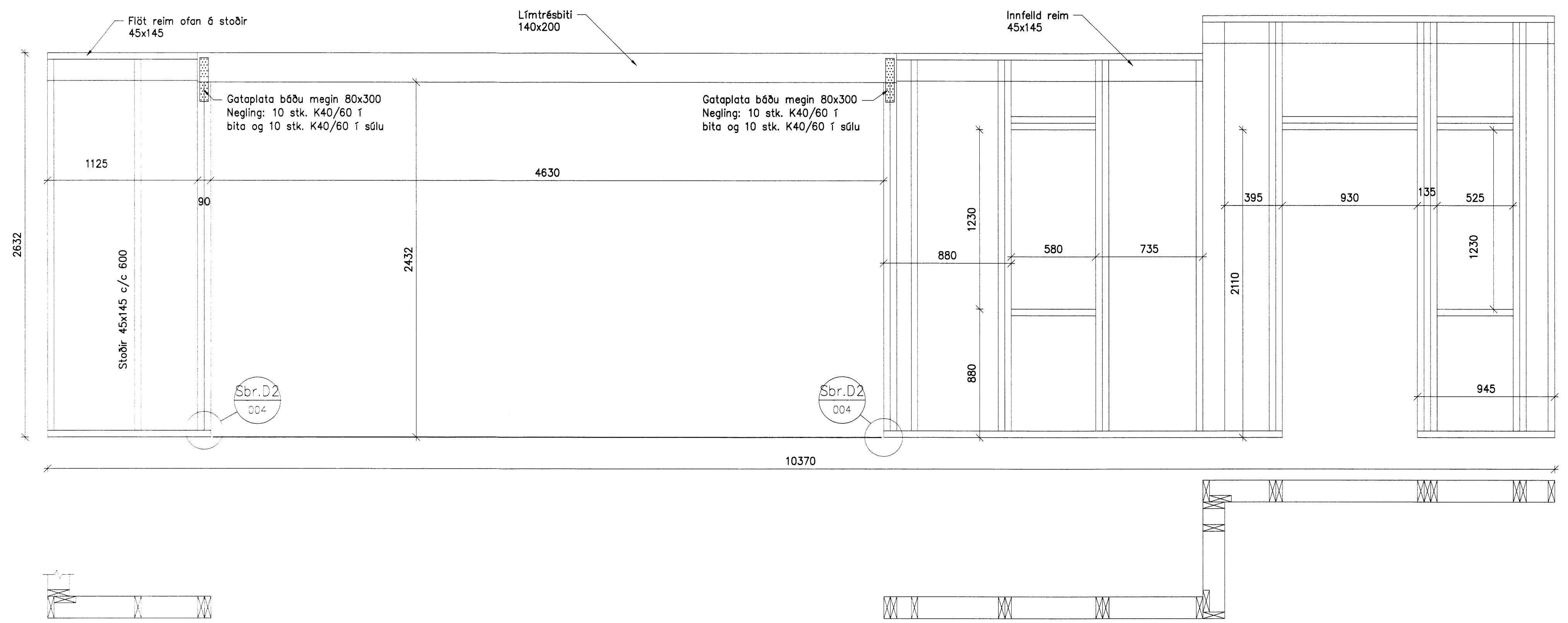
B ÁSÝND 001 1:20
