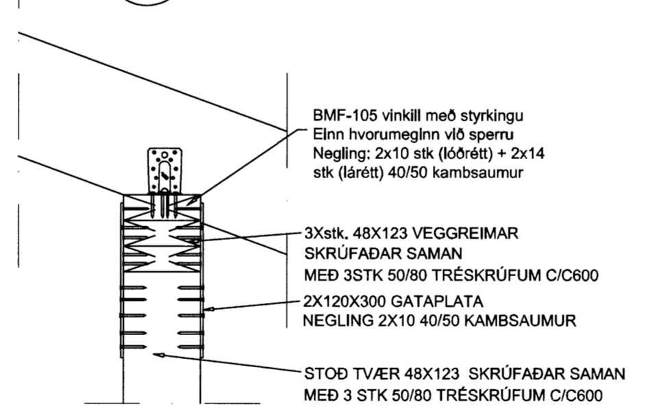
F11 Festing F11 1:10
