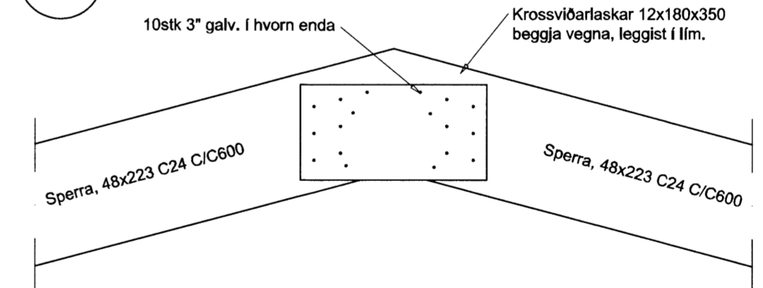
F10 Festing F10 1:10
