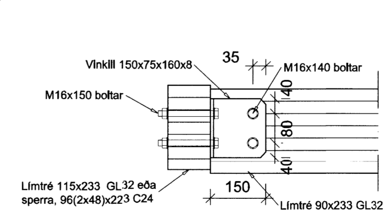
b Snið festing F5 2-1.1 1:10
