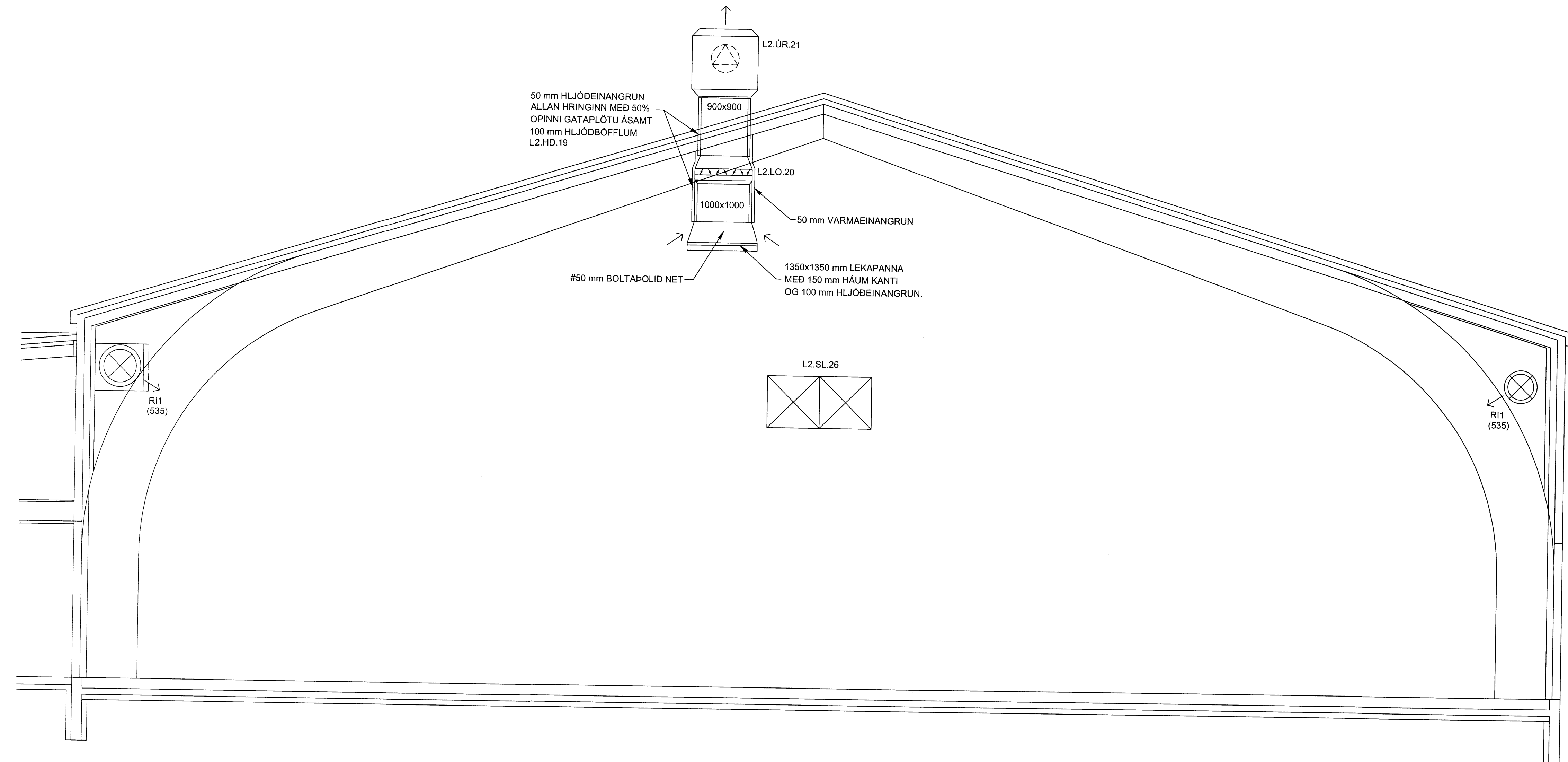
SNID A - A Mkv. 1:50
