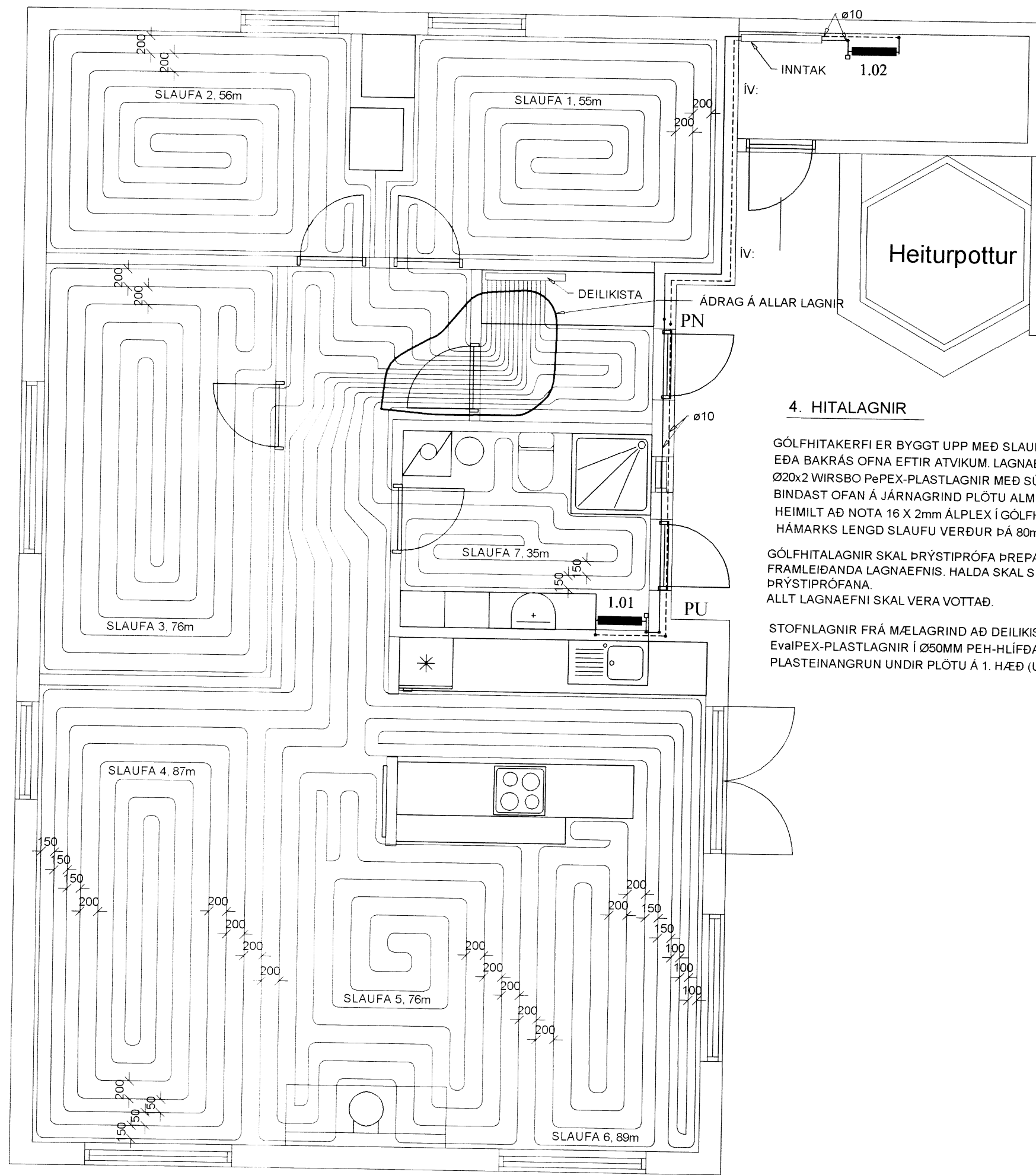
GRUNNMYND GÓLFHITALAGNA, 1:50
