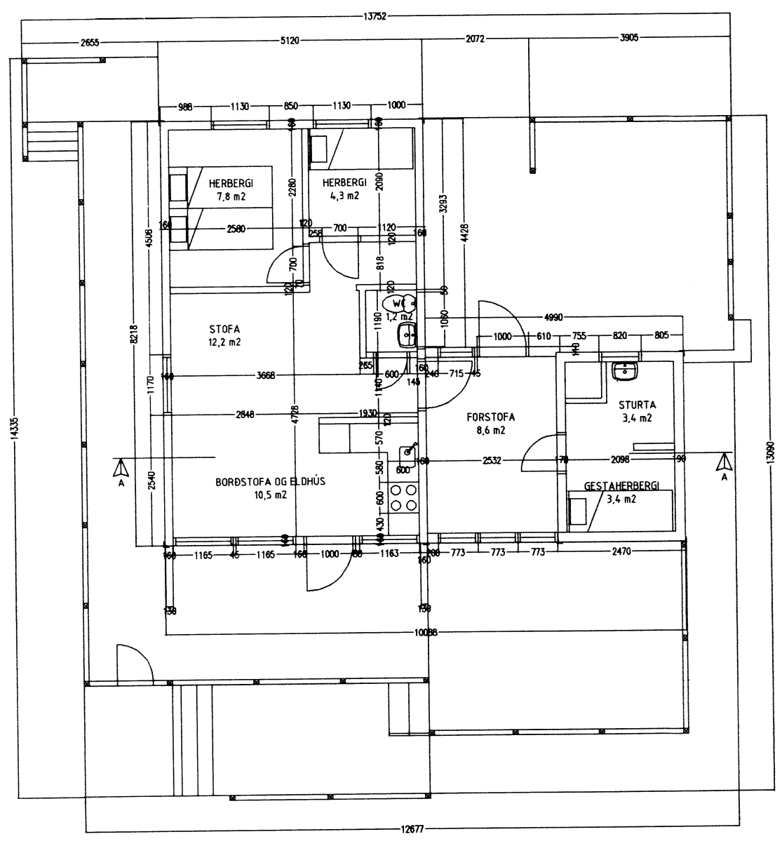
GRUNNMYND 1:100
