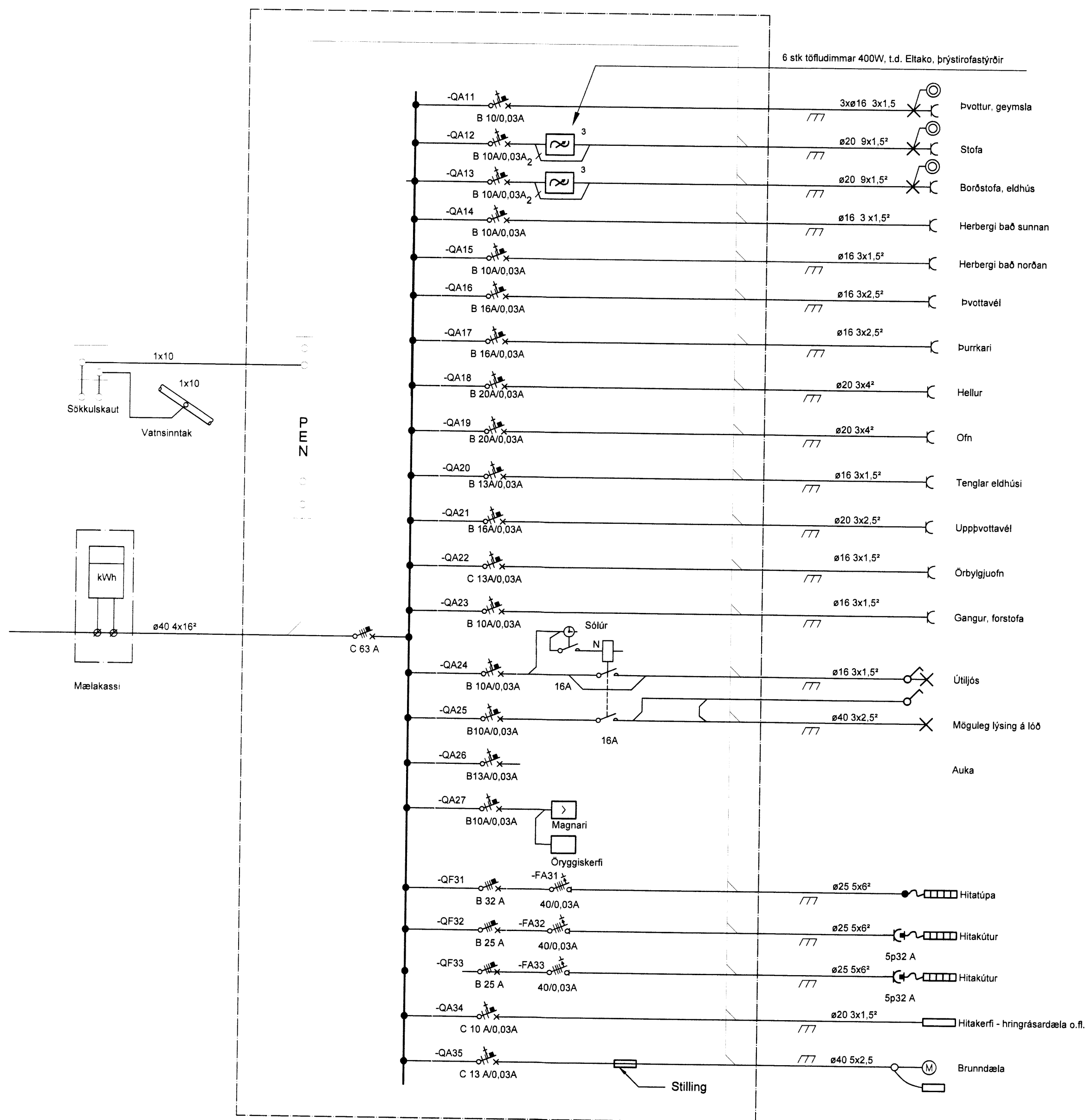
TAFLA -A10 1950x550x205 (HxBxD)með 50mm sökkli Fyrir bæði lágspennu- og smáspennubúnað
