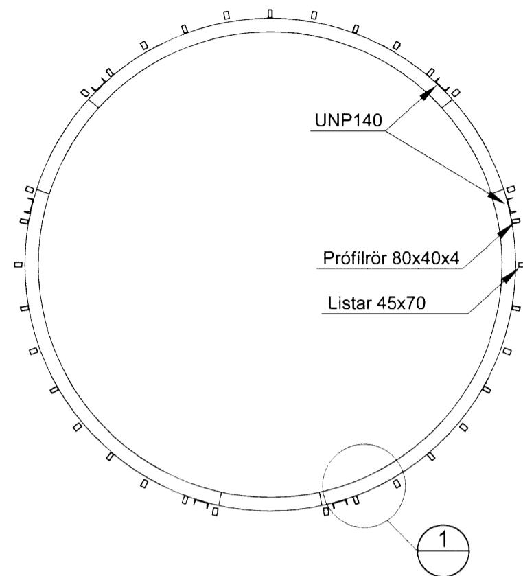
Grunnmynd - Stálstoðir M 1:50
