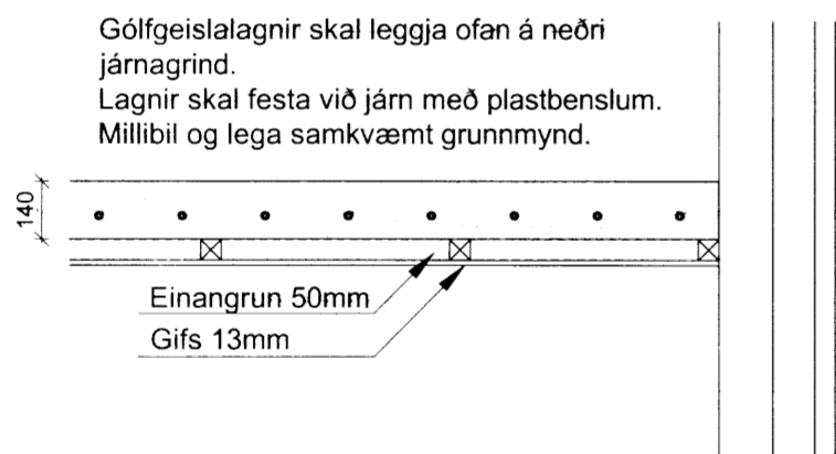
A Snið í gólplötu 1:20
