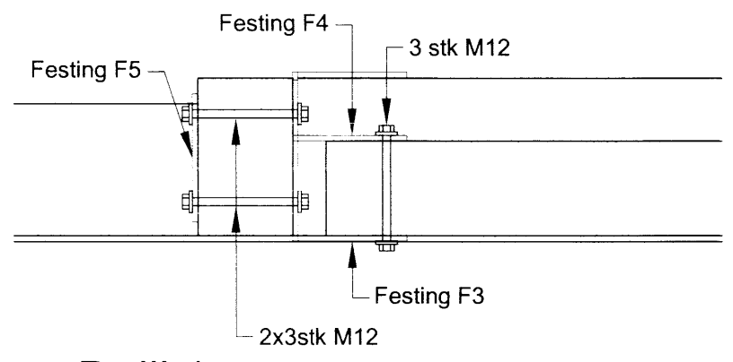
Deili 1 M 1:10
