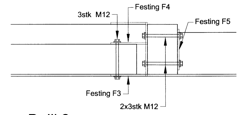
Deili 2 M 1:10
