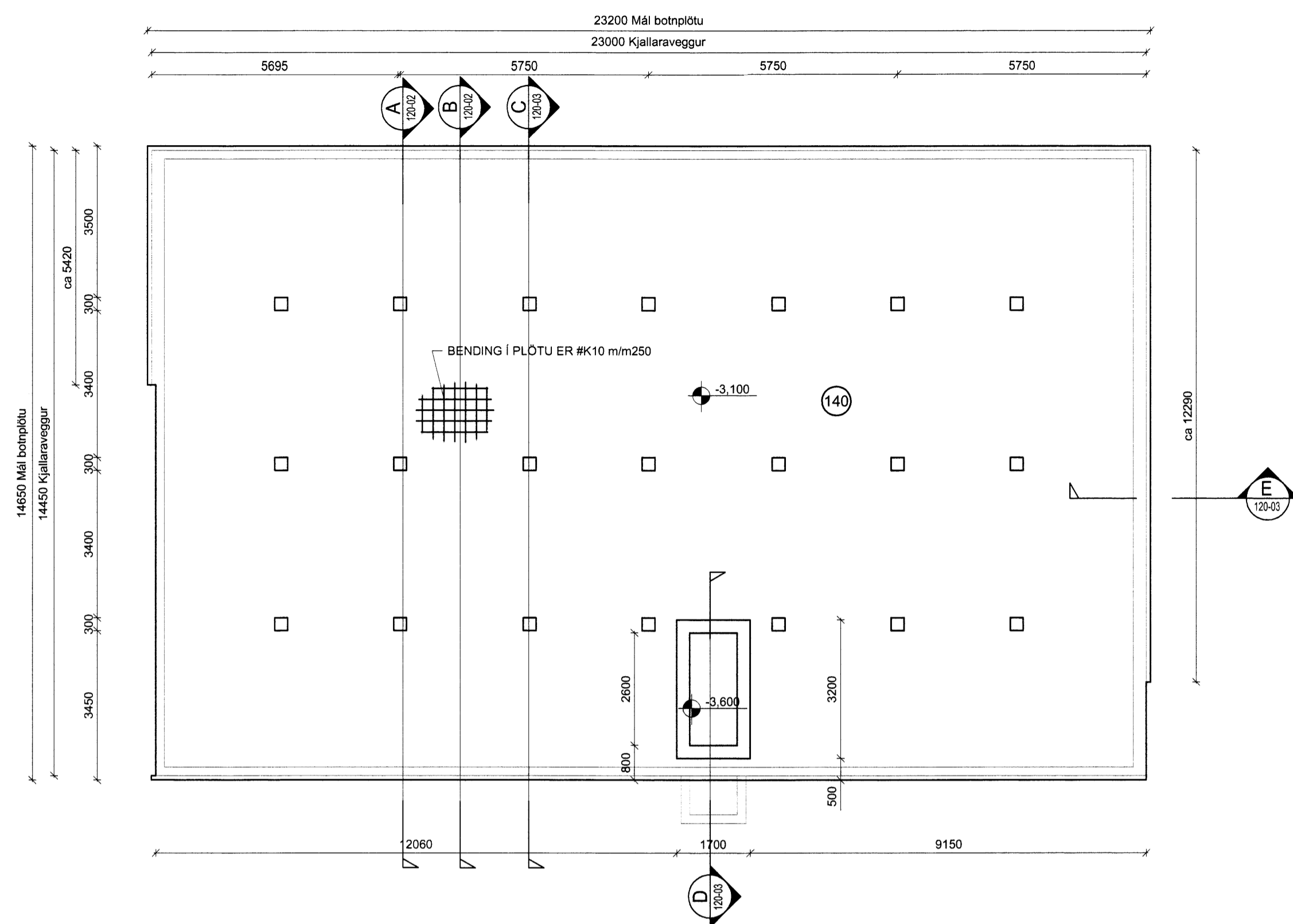
Grunnmynd haugkjallara M 1:100
