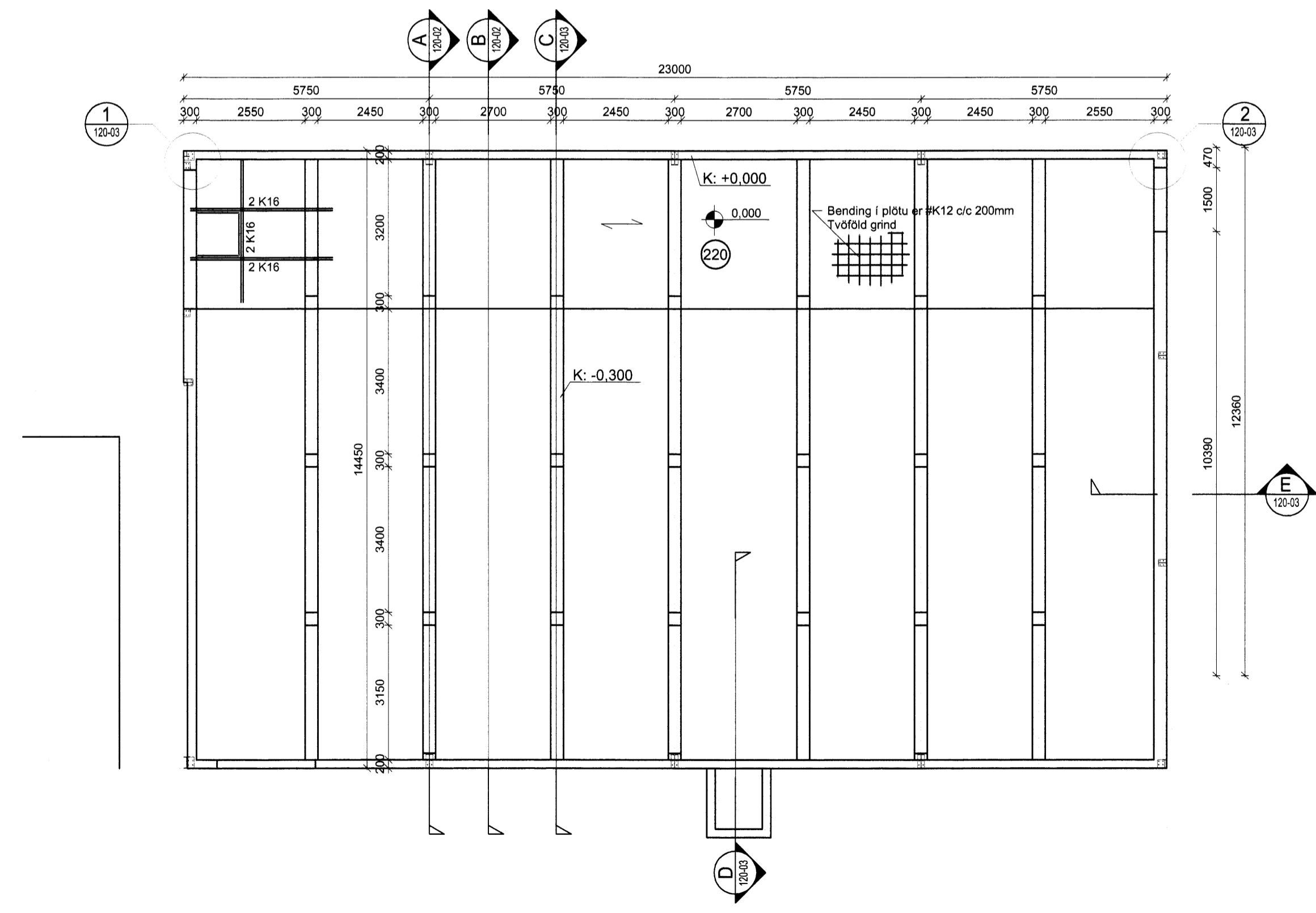
Grunnmynd jarðhæðar M 1:100
