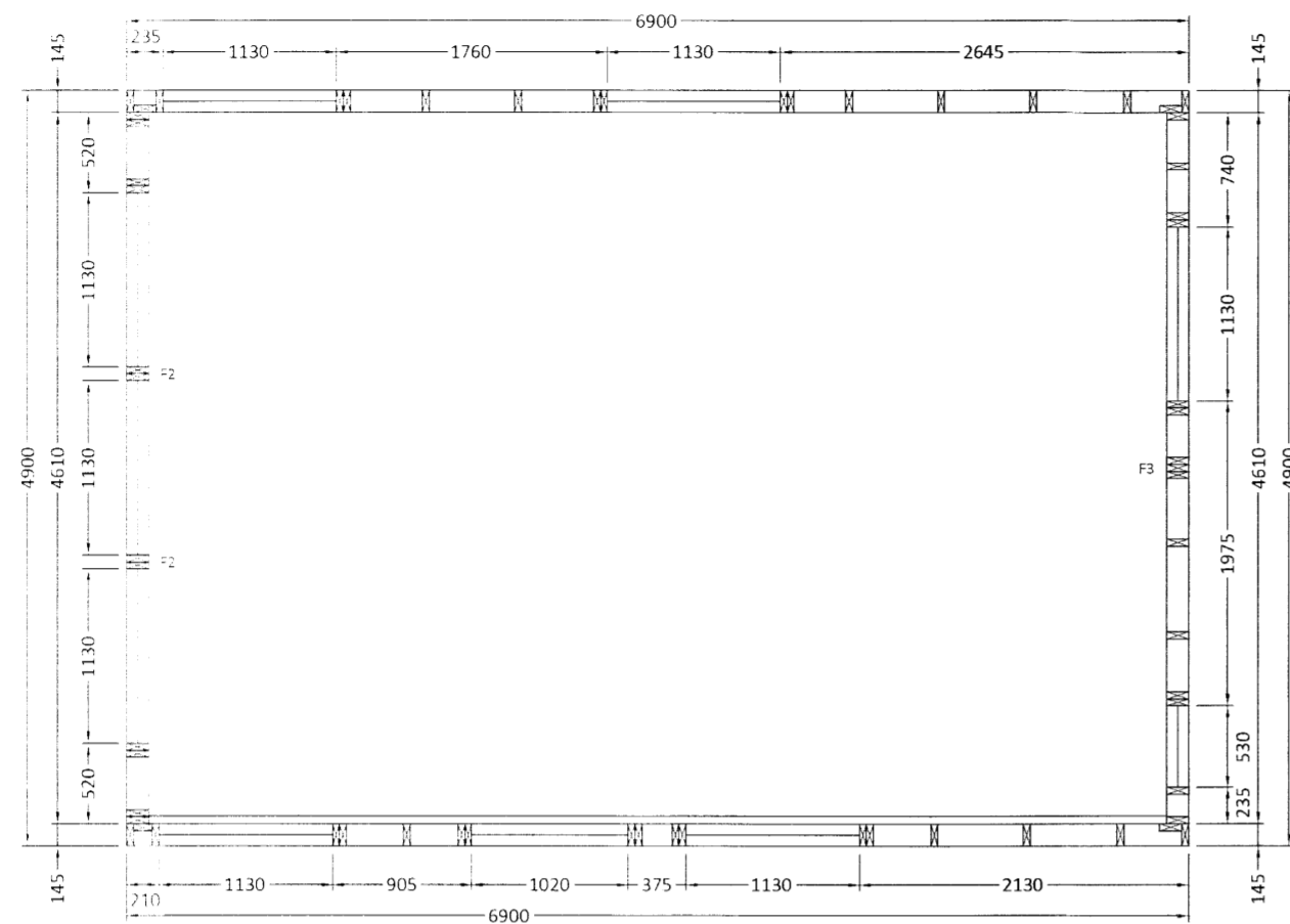
GRUNNMYND VEGGJA MVK. 1:50
