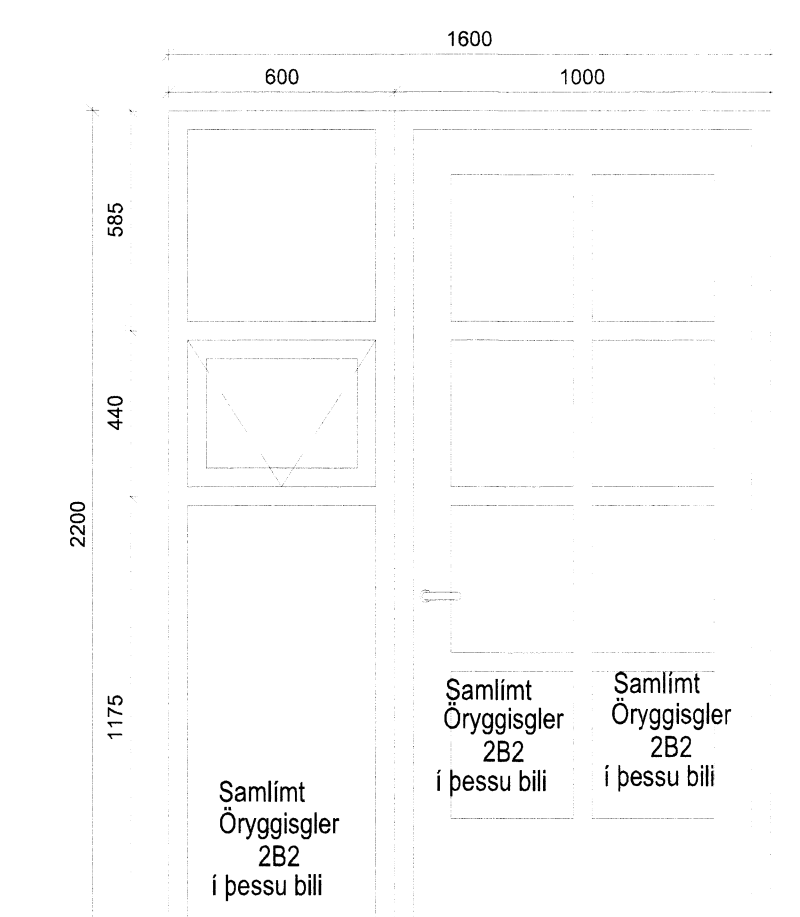
UH 02 7.stk Ásýnd/ Grunnmynd 1:20
