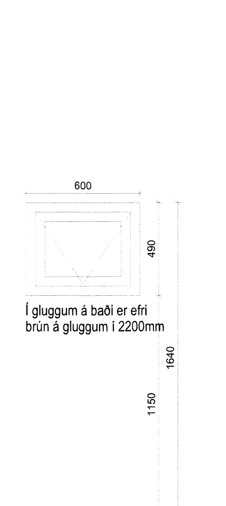
GL 02 4.stk Ásýnd/ Grunnmynd 1:20
