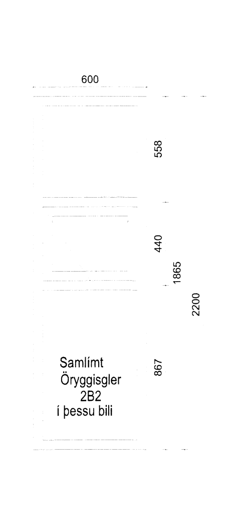
GL 01 2.stk Ásýnd/ Grunnmynd 1:20
