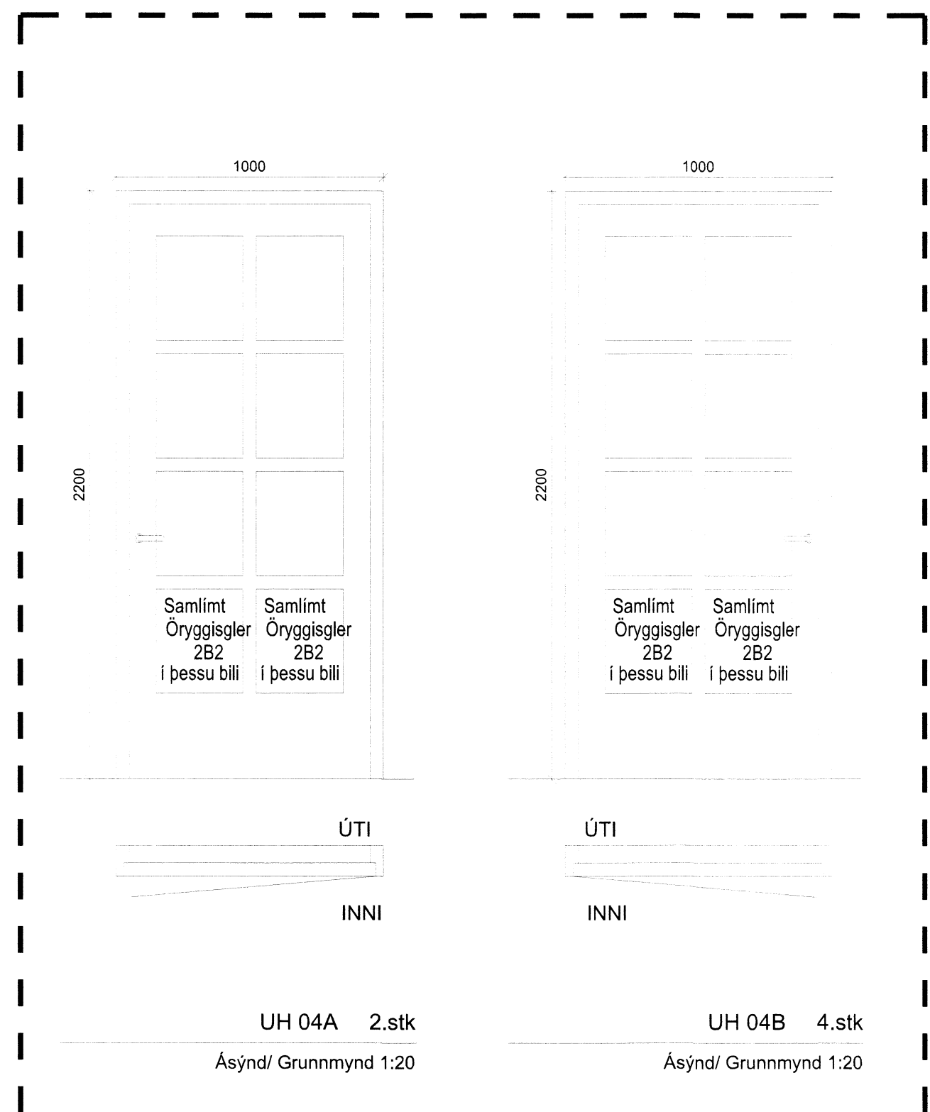
UH 04A 2.stk Ásýnd/ Grunnmynd 1:20 UH 04B 4.stk Ásýnd/ Grunnmynd 1:20 ÞESSAR HURÐIR OPNAST INN - ALLAR ADRAR HURÐIR OPNAST ÚT
