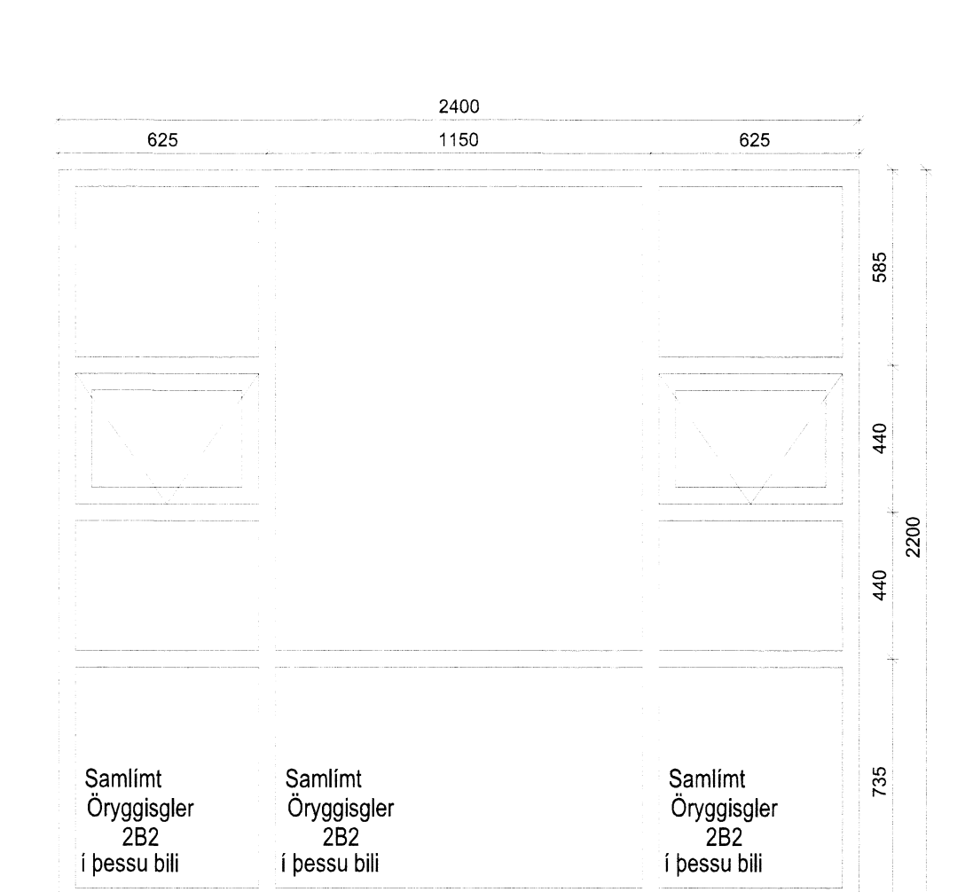
GL 03 6.stk Ásýnd/ Grunnmynd 1:20
