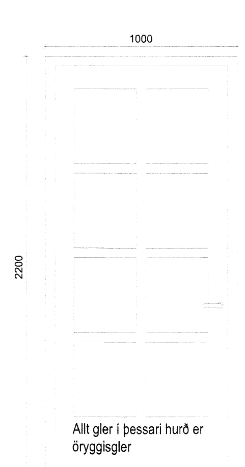
UH 04 1.stk Ásýnd/ Grunnmynd 1:20
