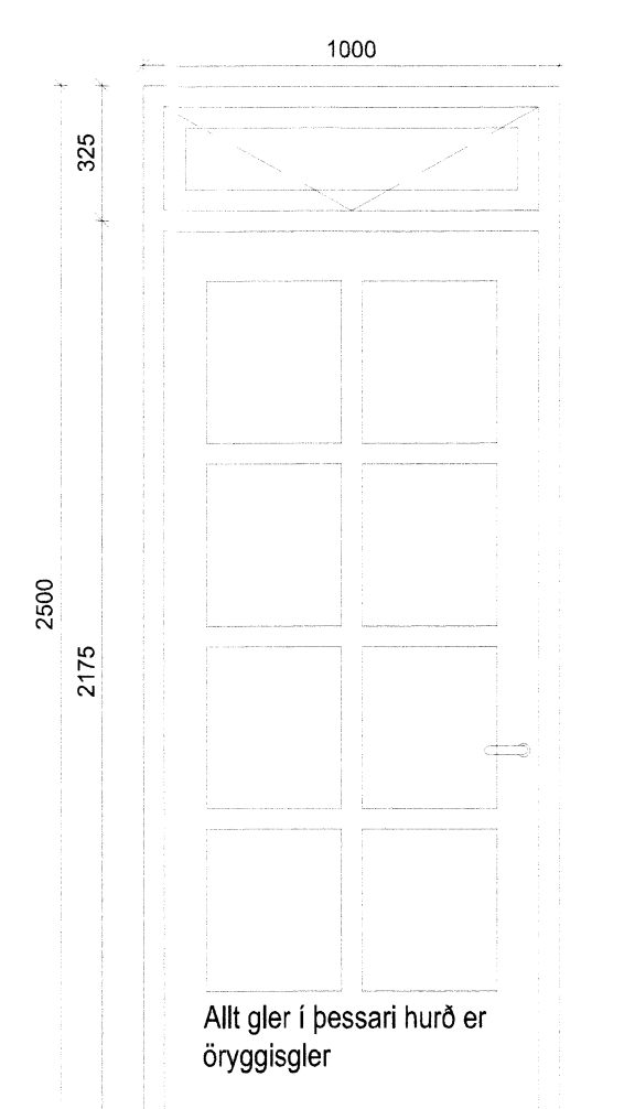
UH 06 1.stk Ásýnd/ Grunnmynd 1:20
