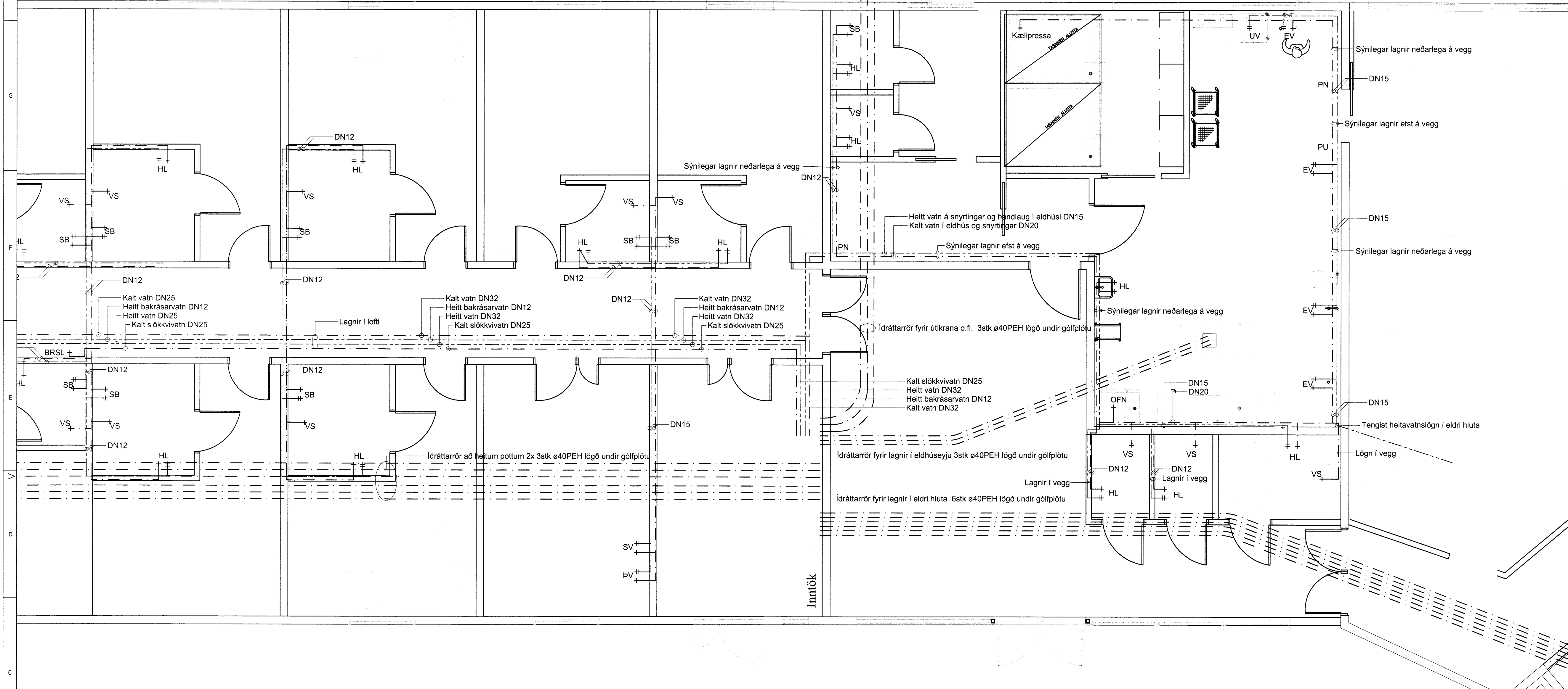
Grunnmynd neysluvatnslagna 1:50
