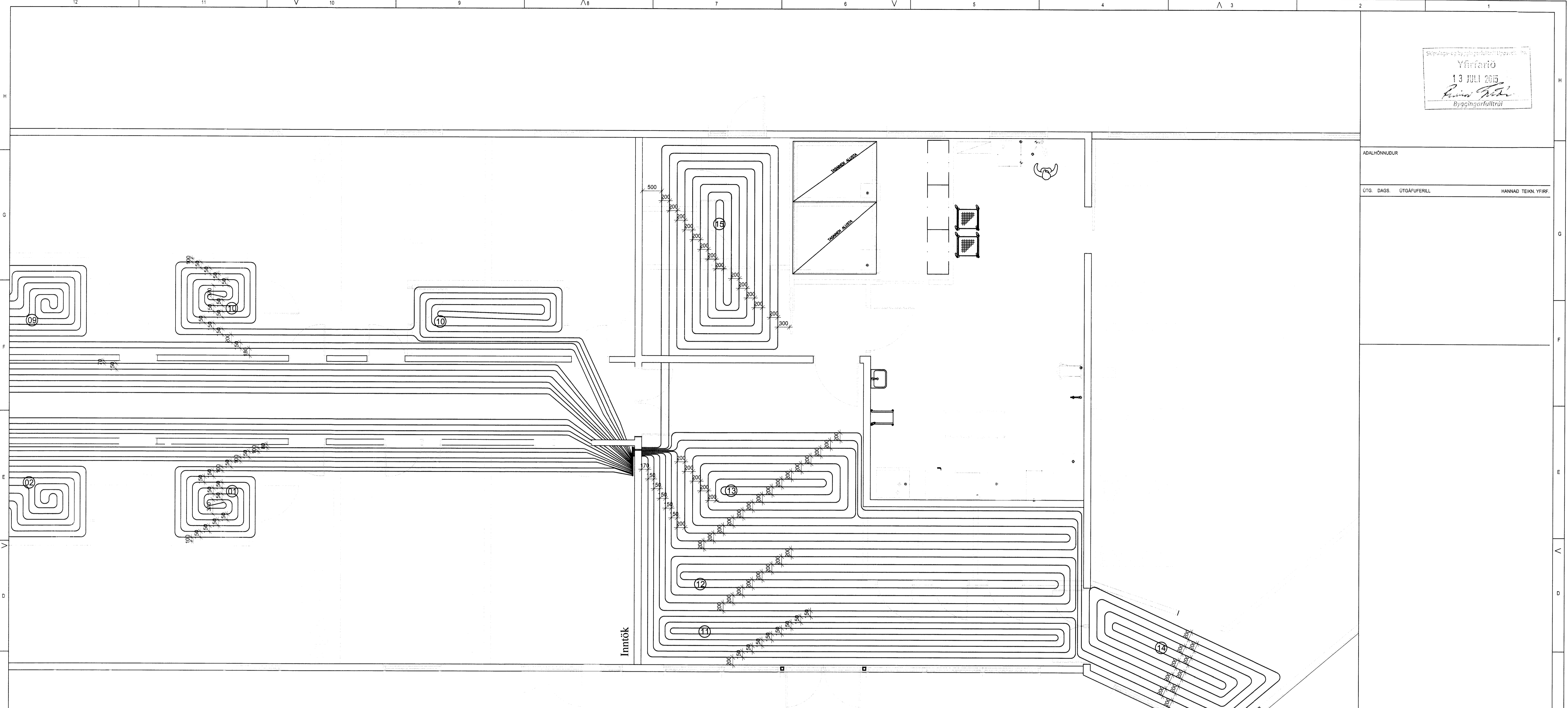
Grunnmynd gólfgeislalagna 1:50
