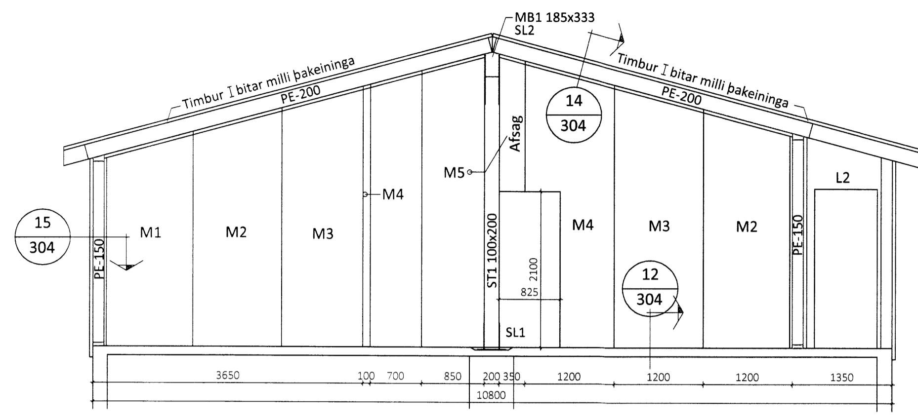
pversnið B-B Mkv. 1:50 301
