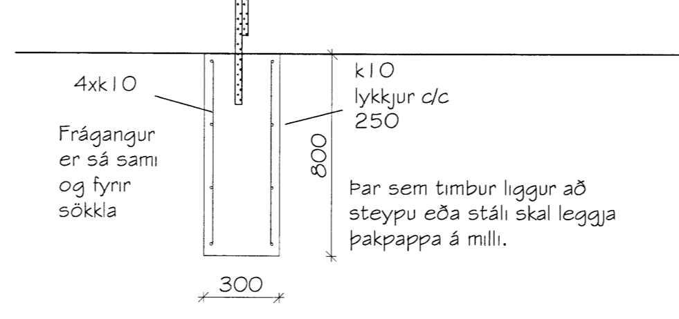
Snið B 1:20
