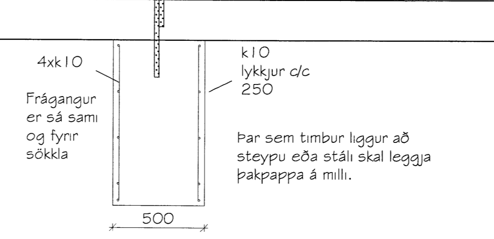
Snið A 1:20
