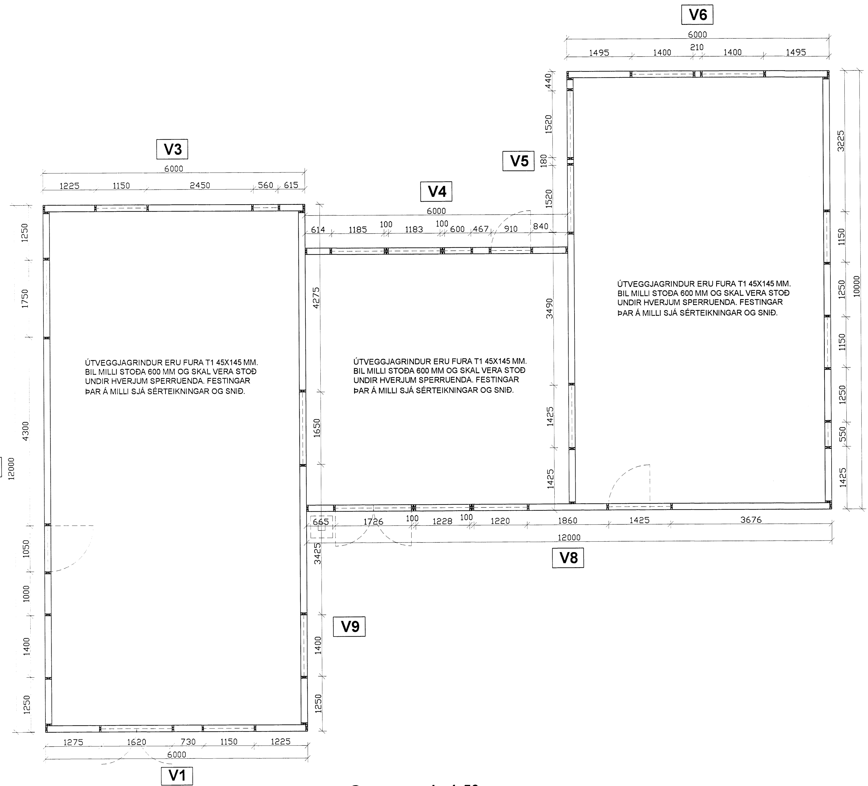
Grunnmynd - 1:50
