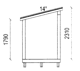
Snið í Geymslu Mkv. 1:100
