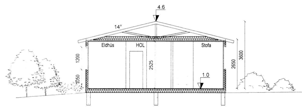
Snið A-A Mkv. 1:100
