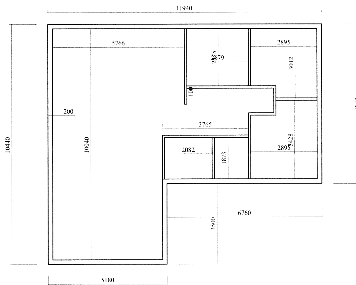
Grunnmynd sökklá 1:100
