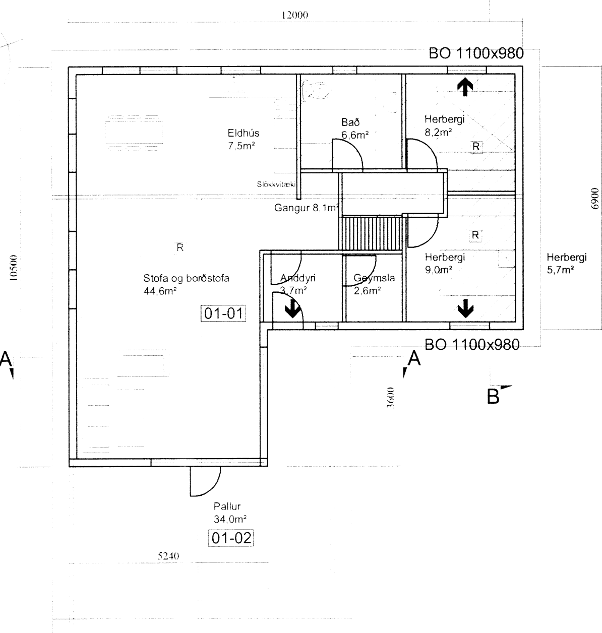
Grunnmynd 1:100
