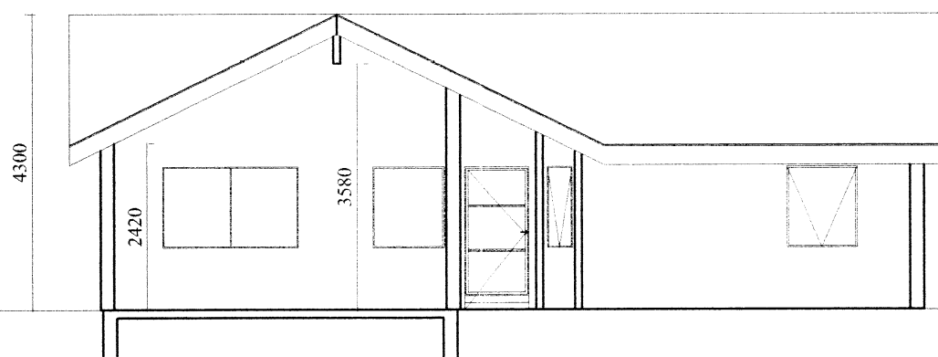
Skurðmynd A-A 1:100
