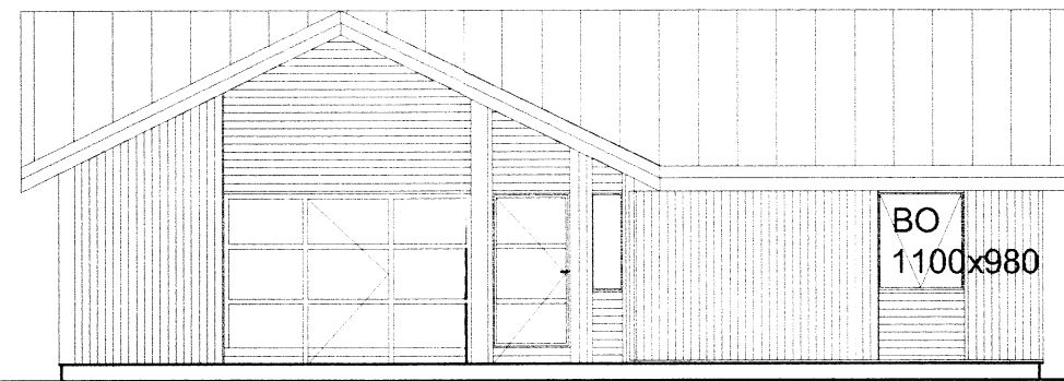
Útlit Suður 1:100
