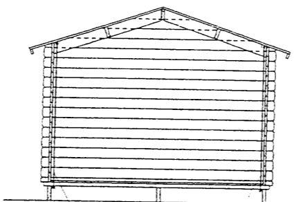
SNÍÐ Í HÚSI 1 : 50
