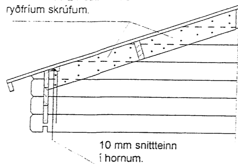
STYRKING Í GAFLI 1 : 20
