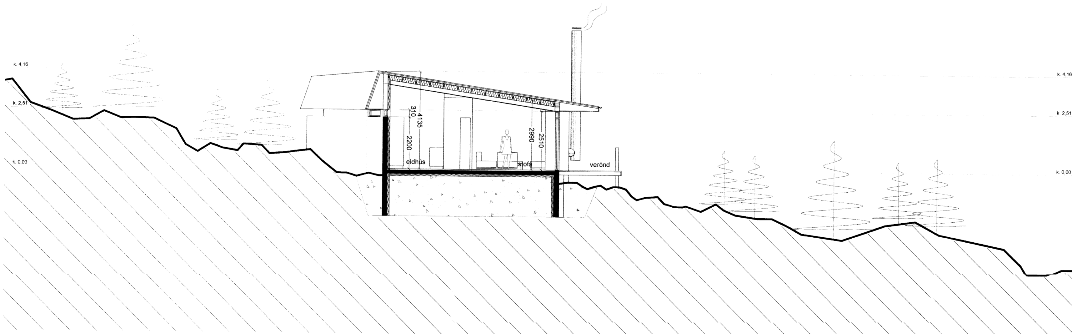
SNEIÐING A - A M 1 : 100
