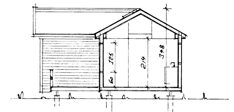
SNEIDMYND A-A.
