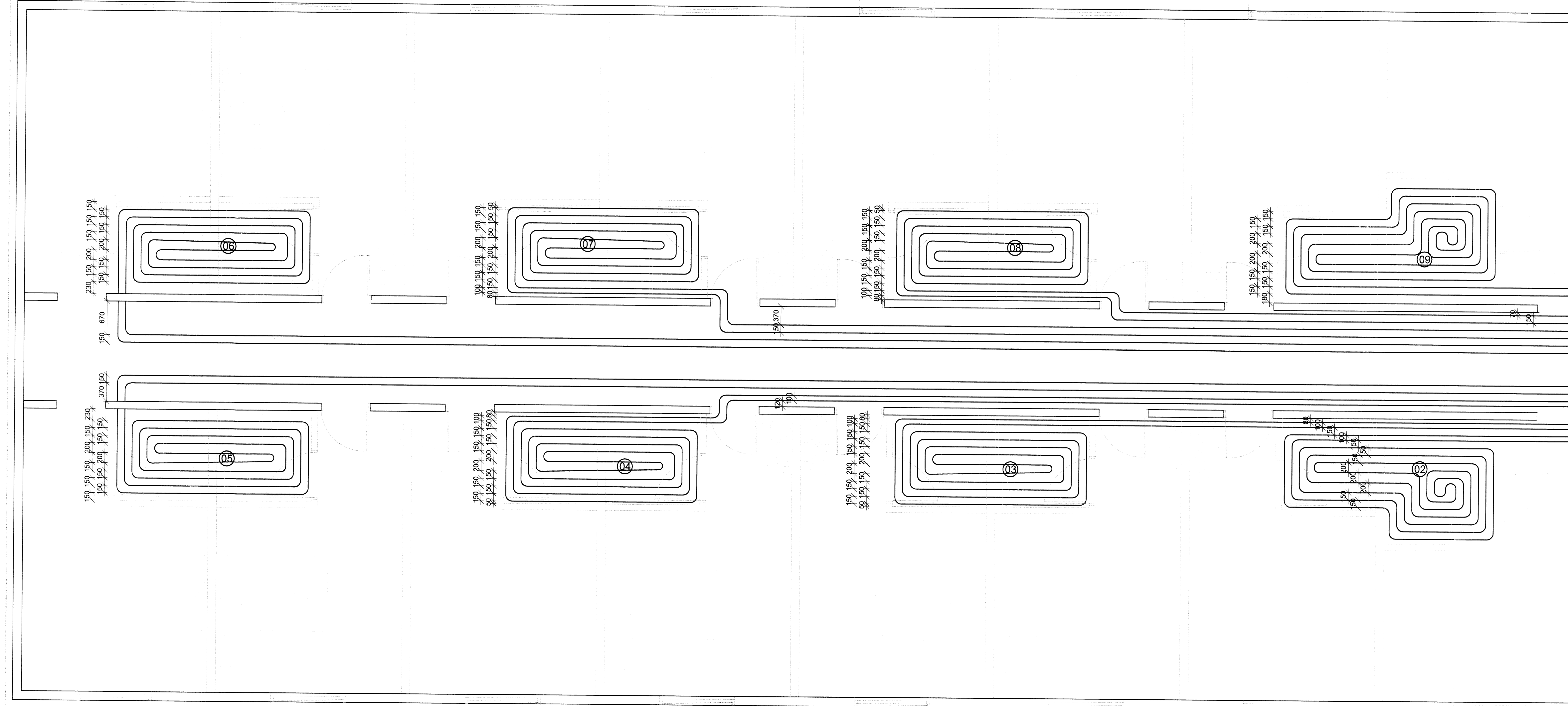
Grunnmynd gólfgeislalagna 1:50
