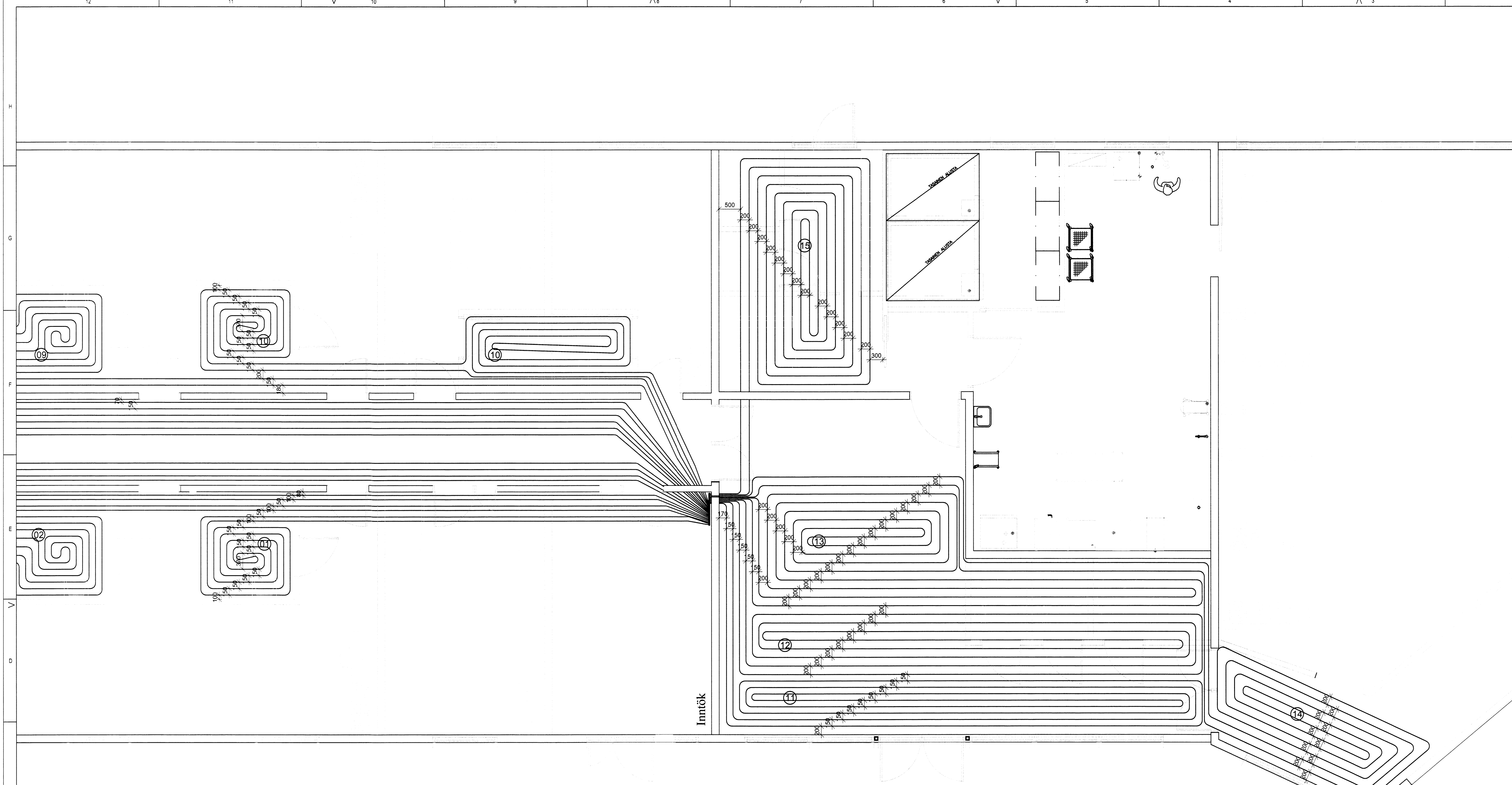
Grunnmynd gólfgeislalagna 1:50
