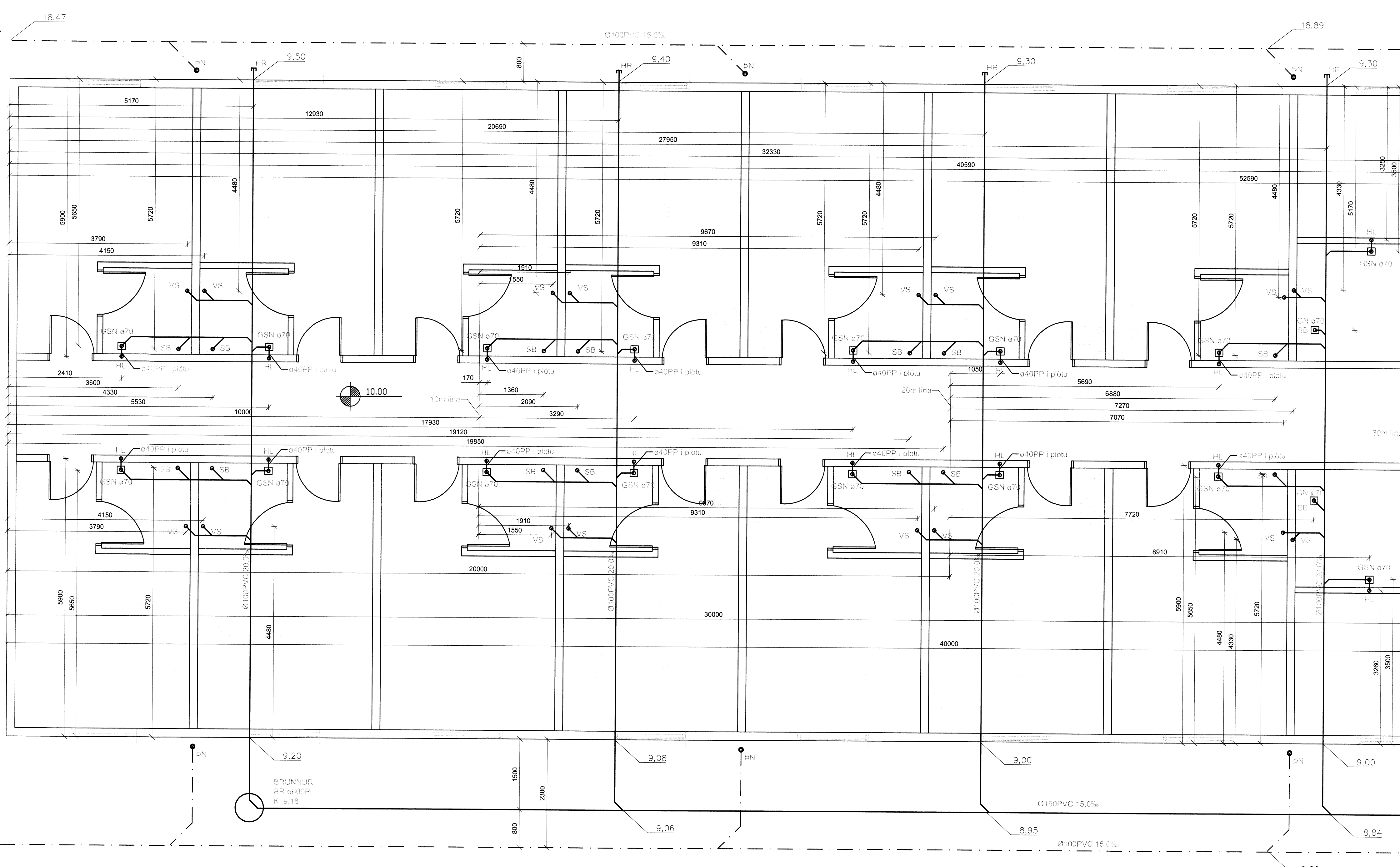
Grunnmynd frænnislagna 1:50
