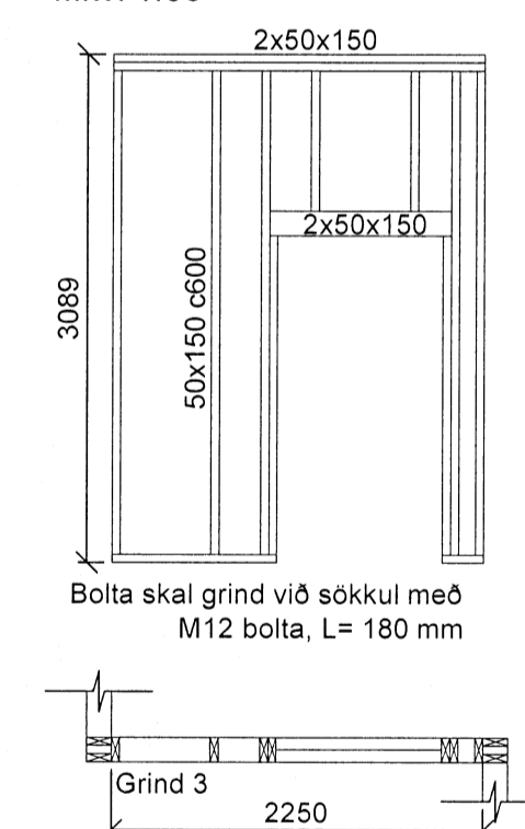
Grind nr. 3 - Sæð utan frá Mkv. 1:50
