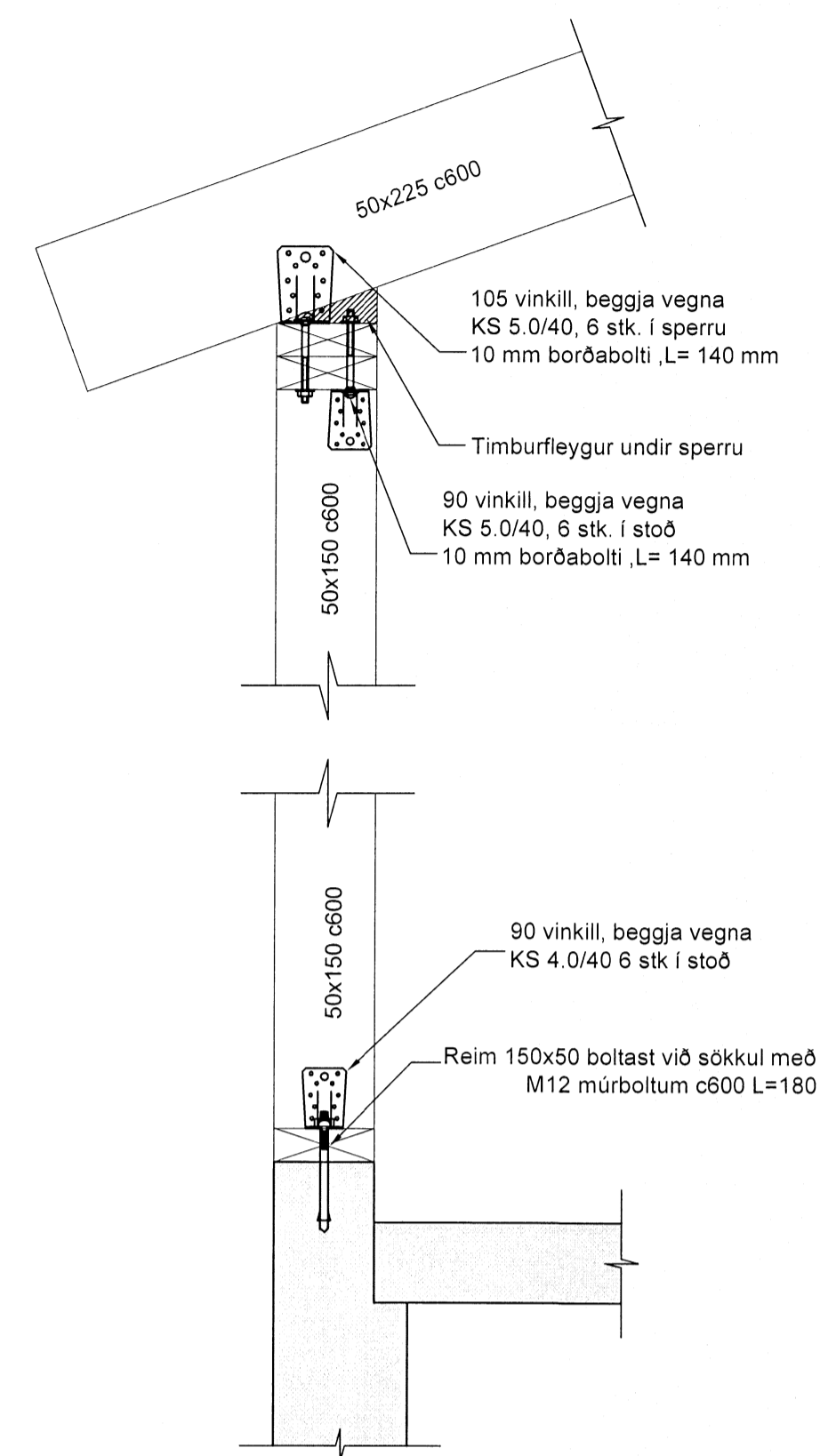
Grind nr. 11 - Sæð utan frá Mkv. 1:50
