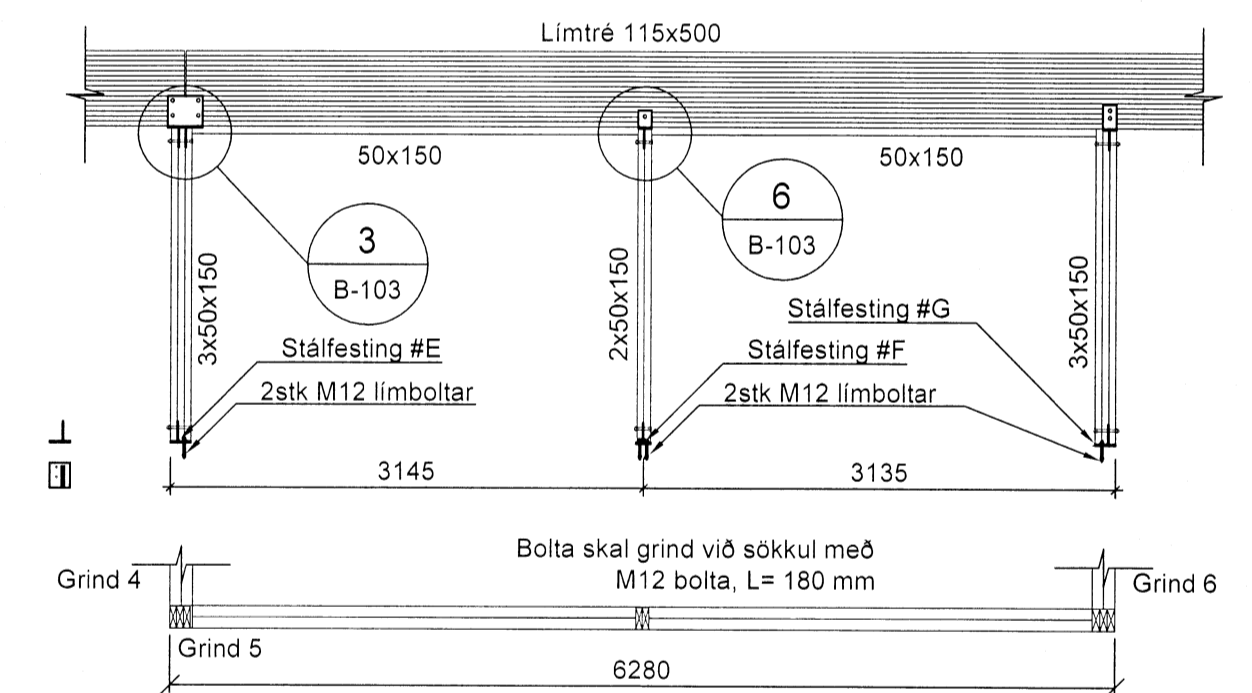
Grind nr. 5 - Sæð utan frá Mkv. 1:50
