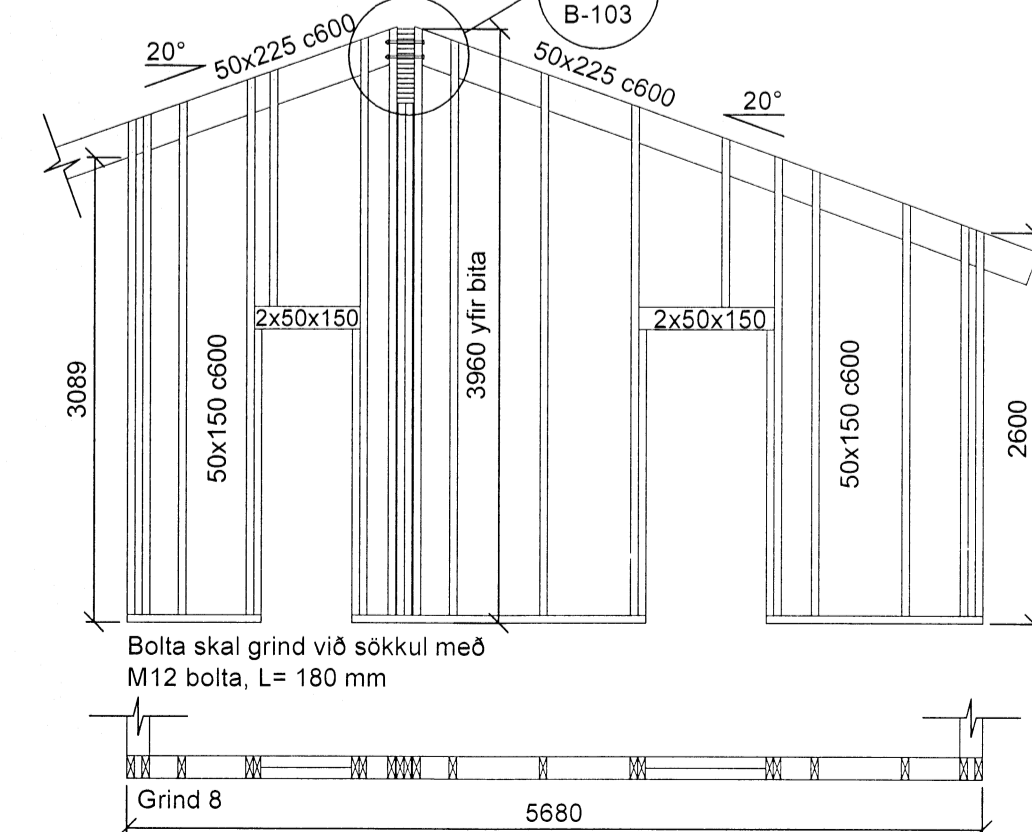
Grind nr. 8 - Sæð utan frá Mkv. 1:50
