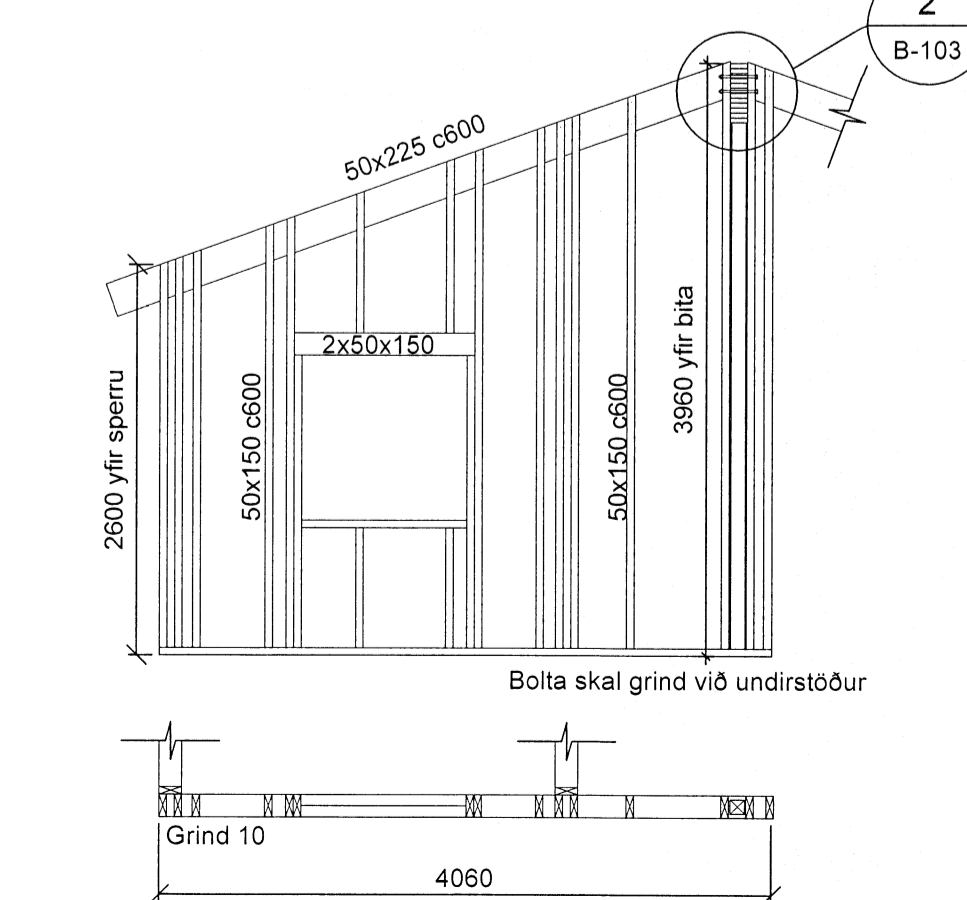
Grind nr. 10 - Sæð utan frá Mkv. 1:50
