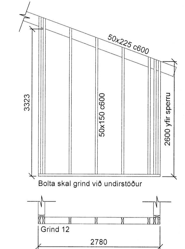
Grind nr. 12 - Sæð utan frá Mkv. 1:50
