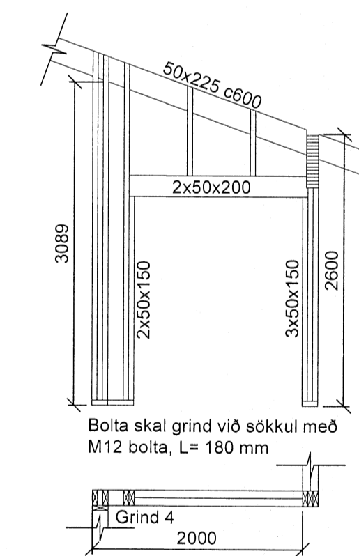
Grind nr. 4 - Sæð utan frá Mkv. 1:50
