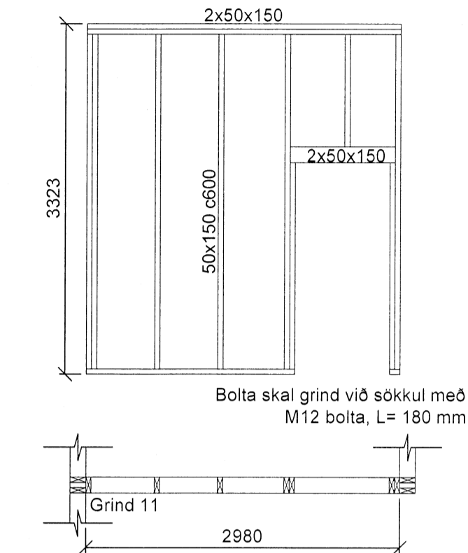
Grind nr. 11 - Sæð utan frá Mkv. 1:50
