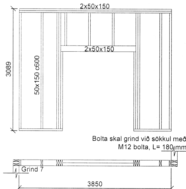
Grind nr. 7 - Sæð utan frá Mkv. 1:50
