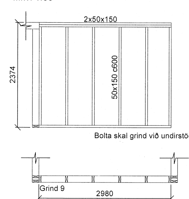
Grind nr. 9 - Sæð utan frá Mkv. 1:50
