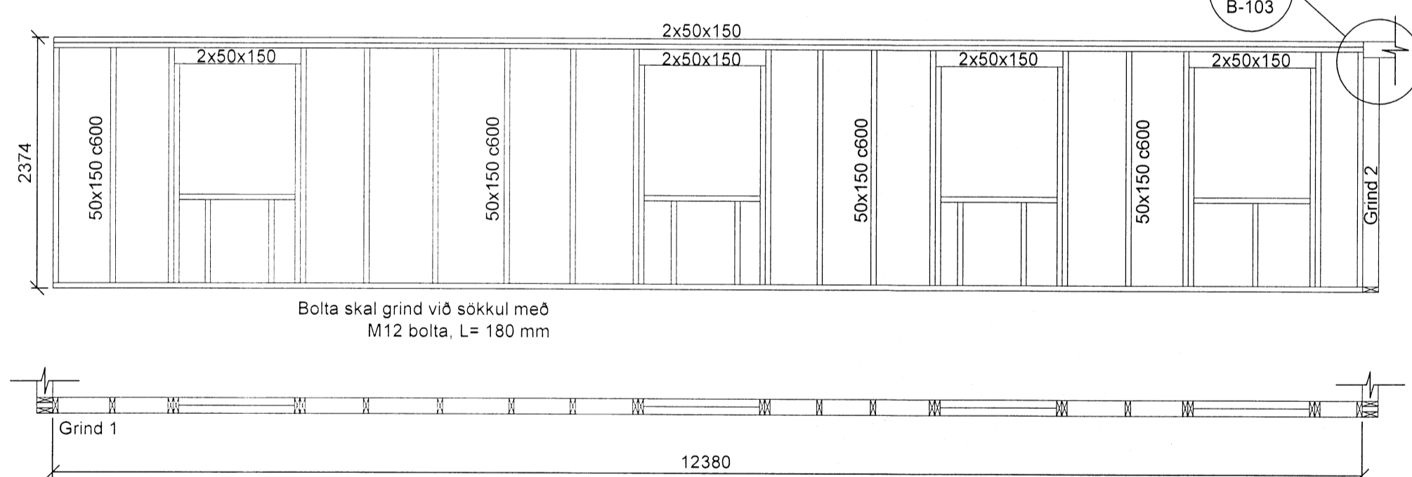
Grind nr. 1 - Sæð utan frá Mkv. 1:50
