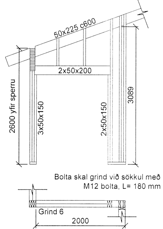
Grind nr. 6 - Sæð utan frá Mkv. 1:50
