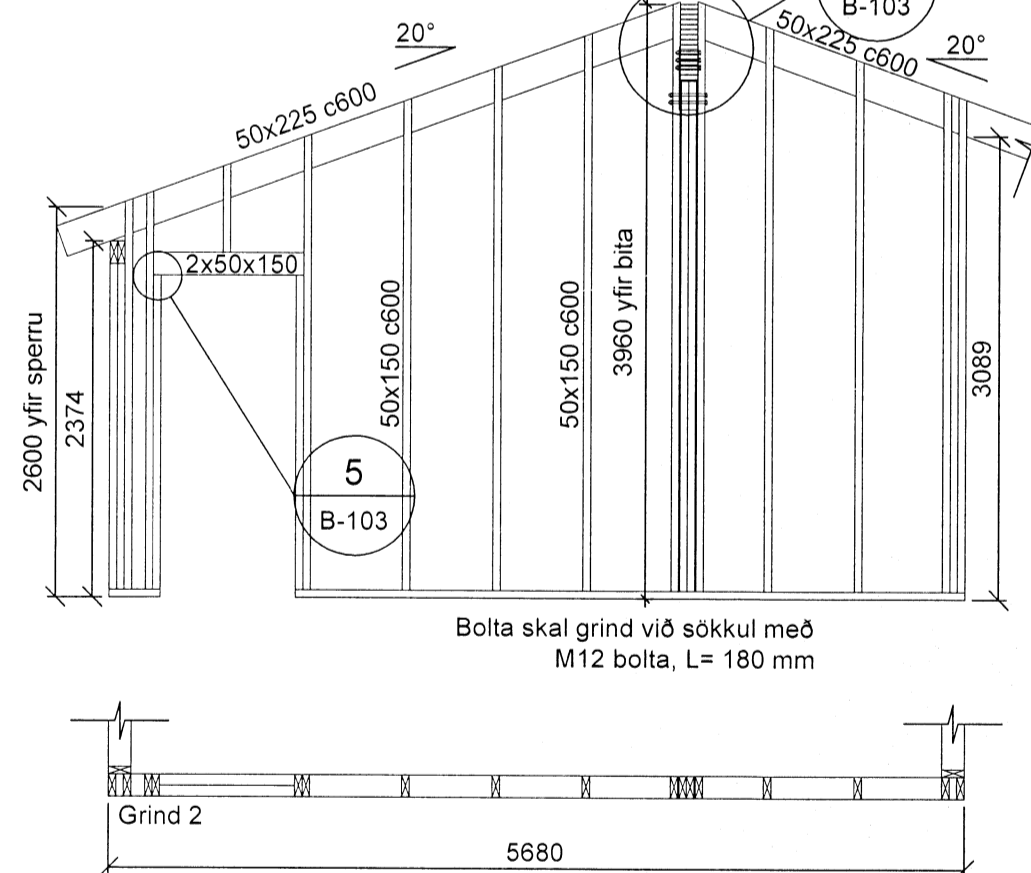
Grind nr. 2 - Sæð utan frá Mkv. 1:50
