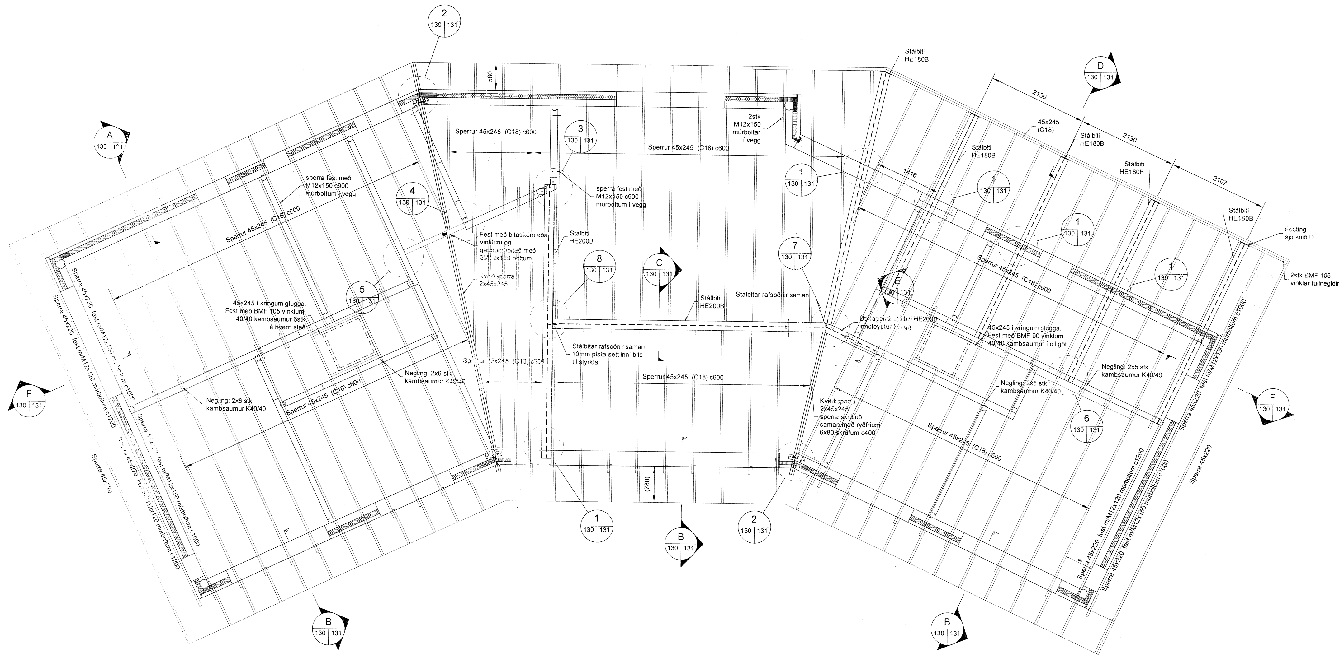
Grunnmynd bakvirkis 1:50
