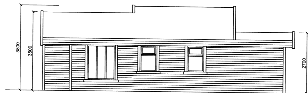
ÚTLIT AUSTUR
