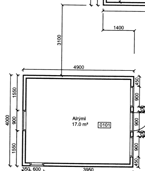
GRUNNMYND GESTAHÚS
