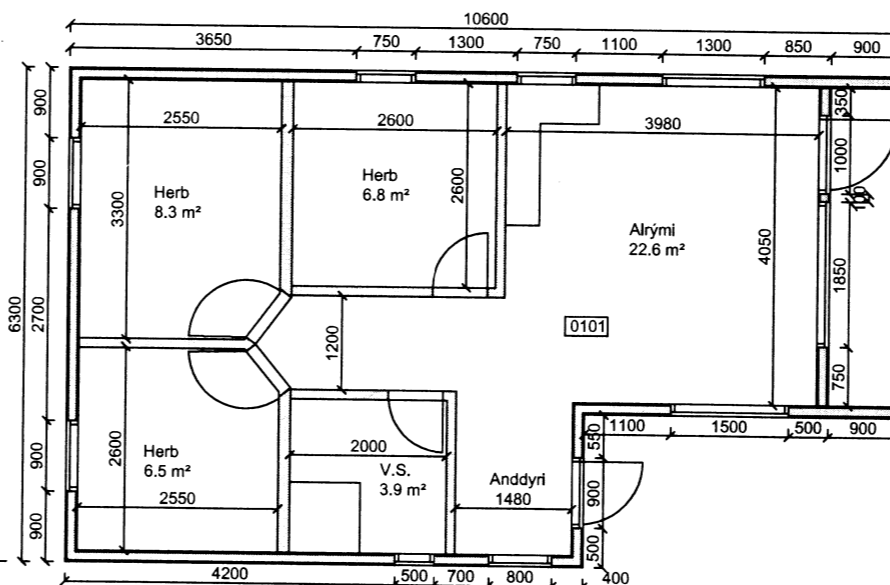
GRUNNMYND HEILSÁRSHÚS
