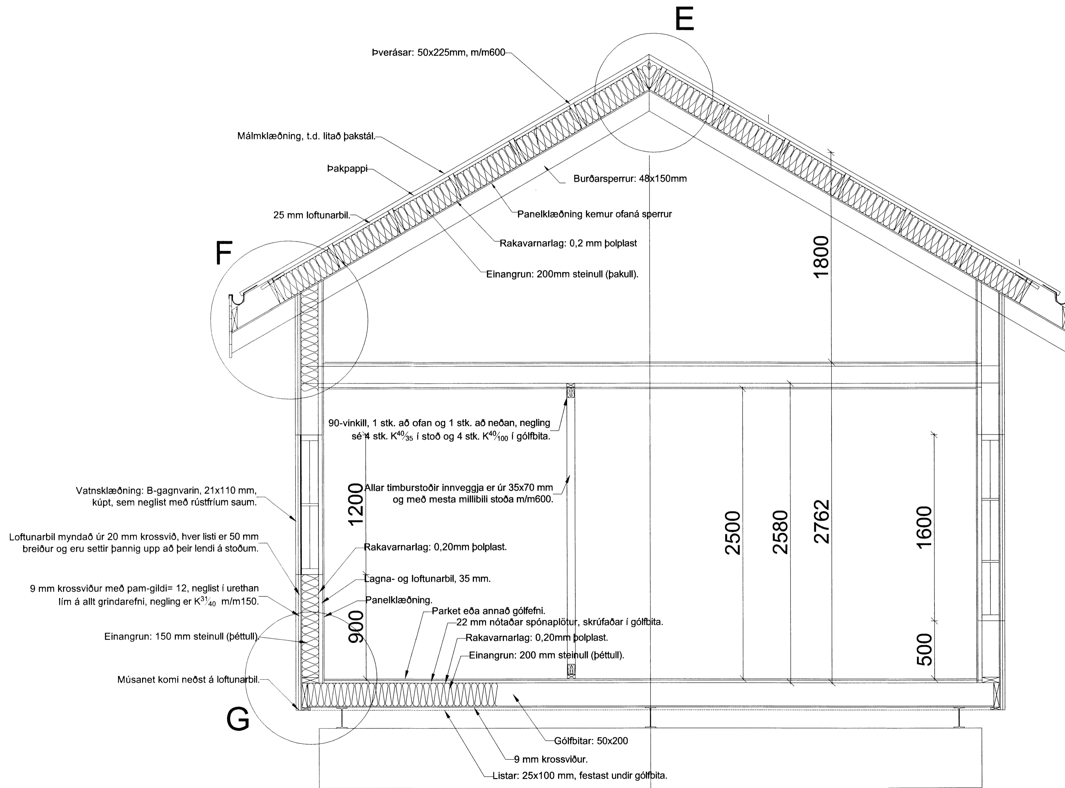
Kennisnið í sumarbústað með efnisskýringum, mkv.= 1:20.
