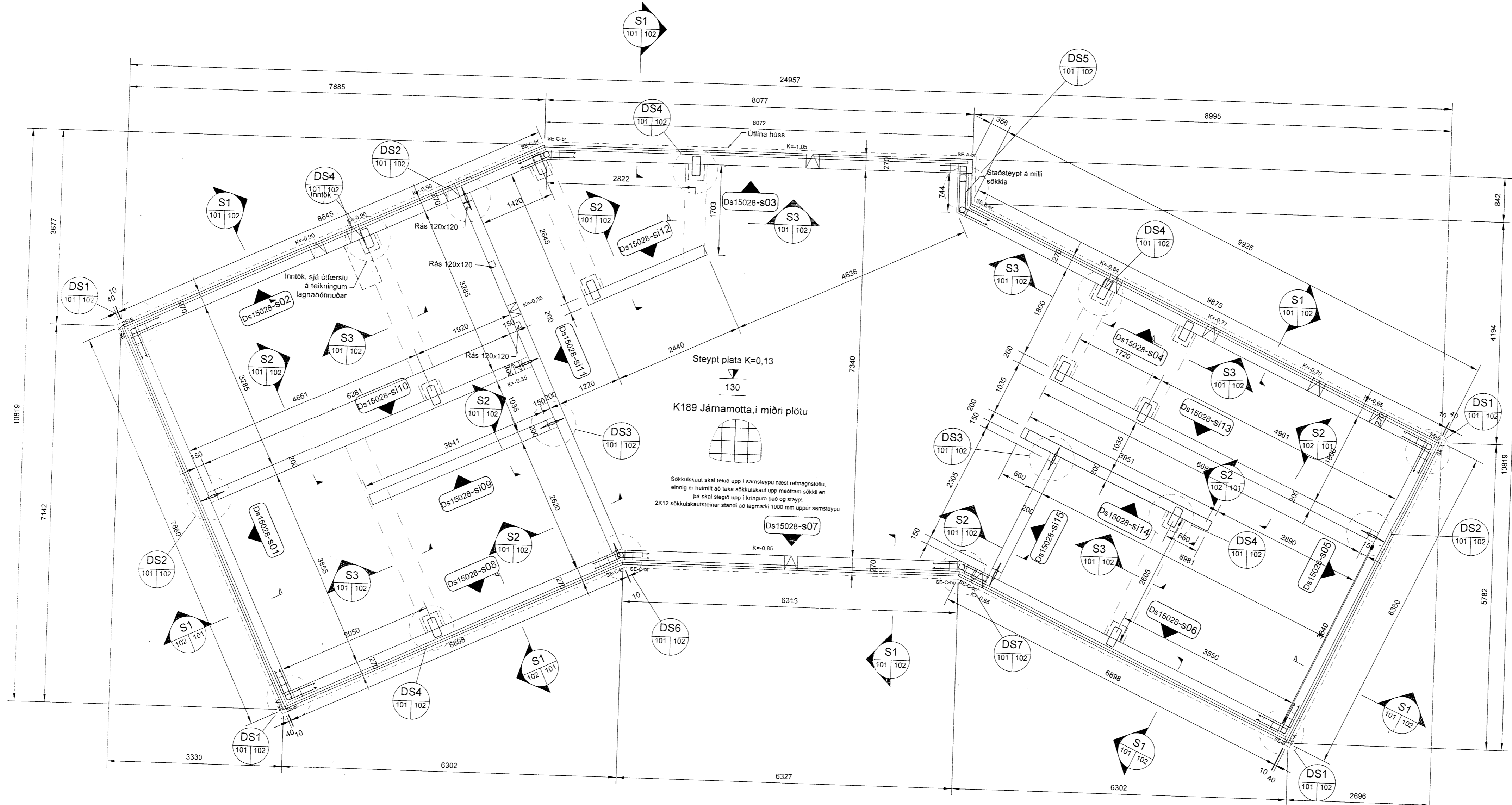
Grunnmynd sökklar 1:50
